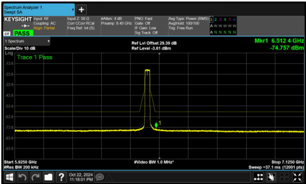
Figure 353 - A (Core 0) 802.11ax HE20 SU LPI 6475 MHz (CH105)
