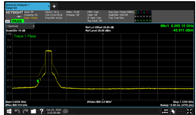
Figure 357 - A (Core 0) 802.11ax HE40 SU SP 6165 MHz (CH43)
