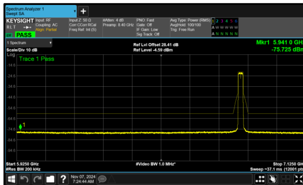
Figure 348 - B (Core 1) 802.11ax HE20 SU VLP 6855 MHz (CH181)
