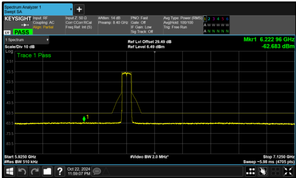
Figure 354 - A (Core 0) 802.11ax HE40 SU LPI 6405 MHz (CH91)
