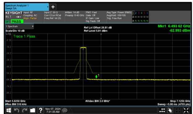
Figure 349 - A (Core 0) 802.11ax HE40 SU VLP 6405 MHz (CH91)
