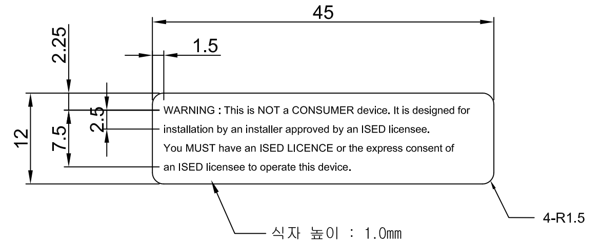
[ RDU용 IC 선언 문구 Label ] [ 4304-001296 ]
