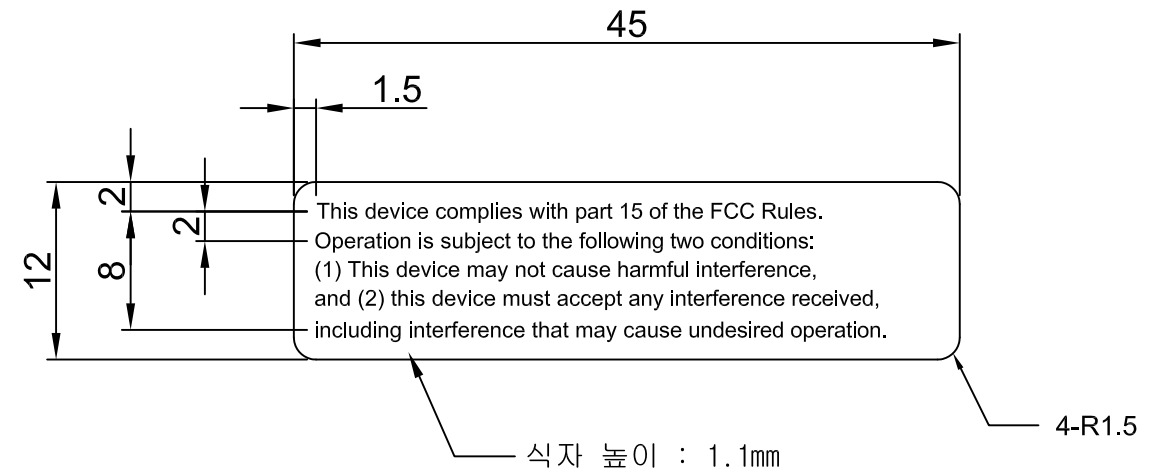
[ HRDU용 FCC 선언 문구 Label ] [ 4304-001064 ]
