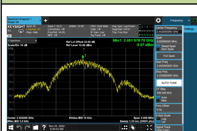
CH00 (2402MHz) LE(1Mbps)
