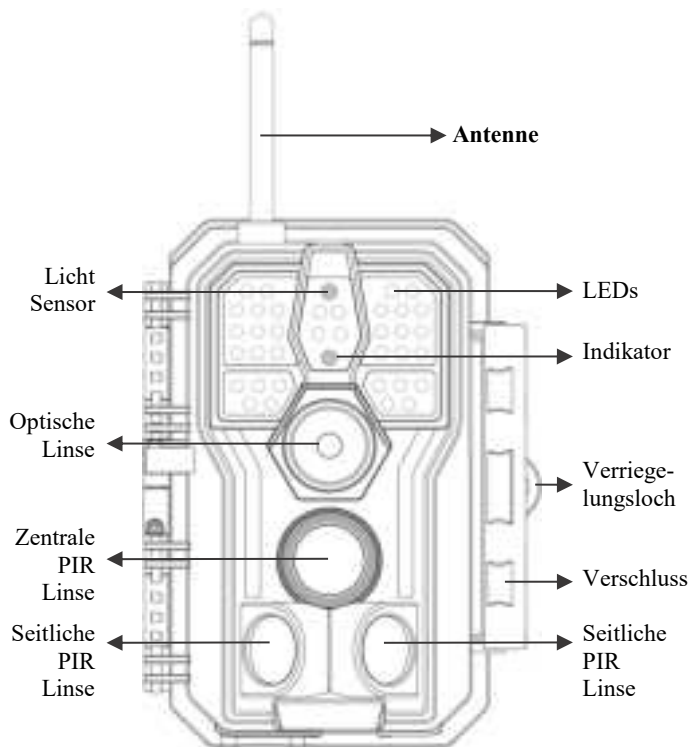
Abb. 1: Vorderansicht
