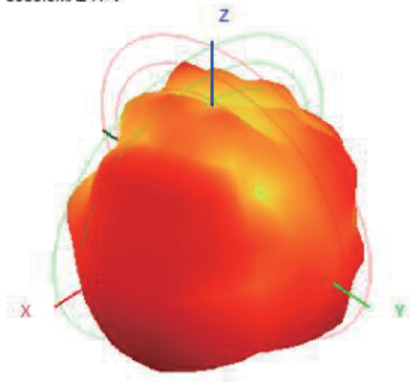
5850.0MHz H+V
