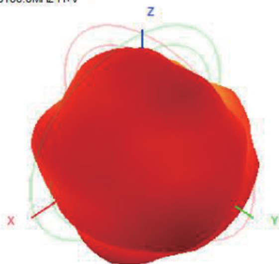
5100.0MHz H+V
