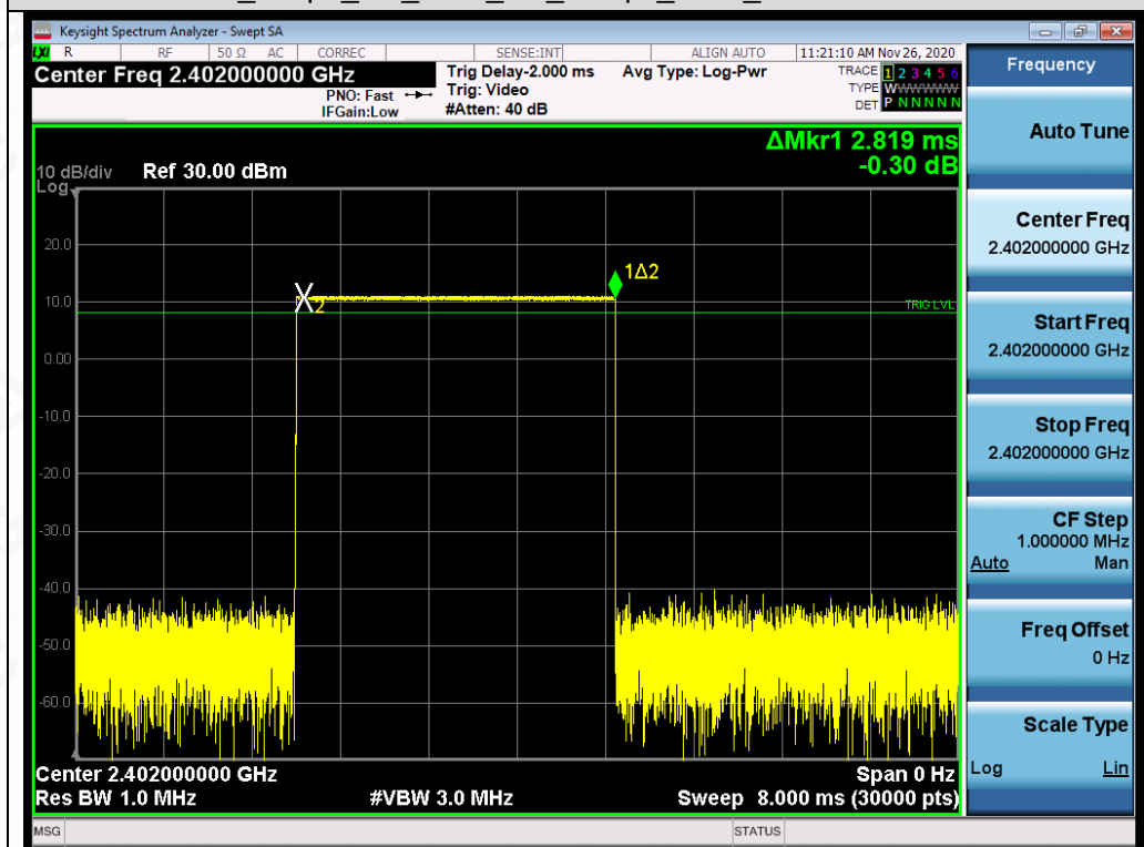
Test_Graph_BR_HOP_NA_1Mbps_2402_Time per Burst
