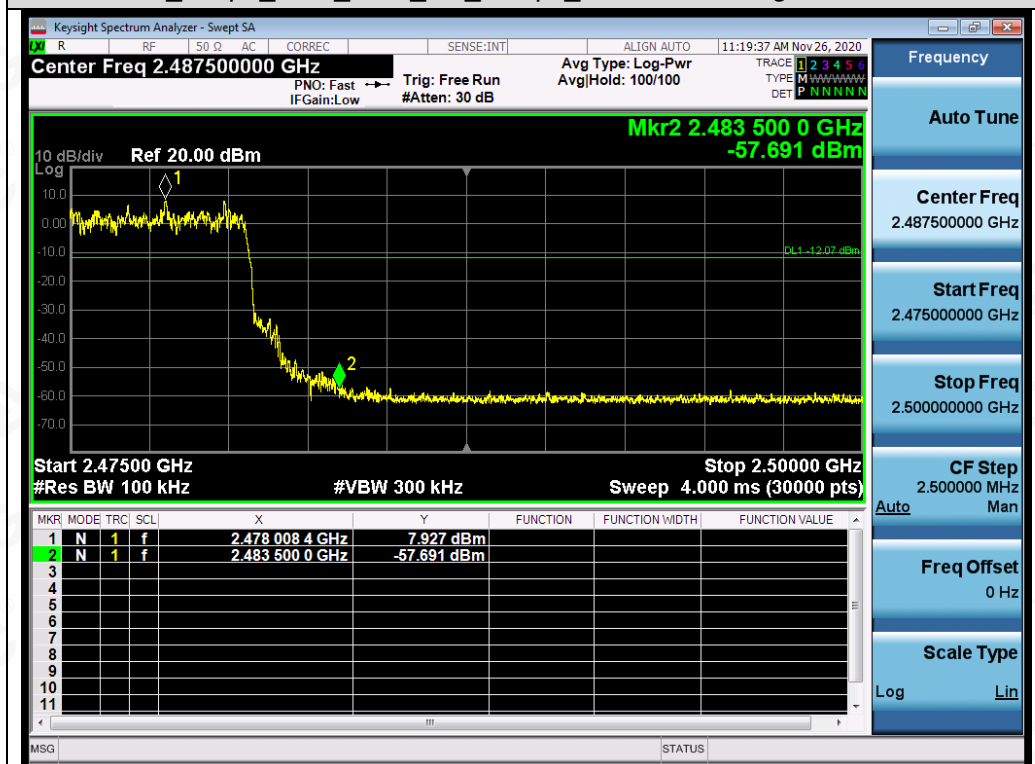
Test_Graph_EDR_HOP_NA_2Mbps_Higher Band Edge Emissions
