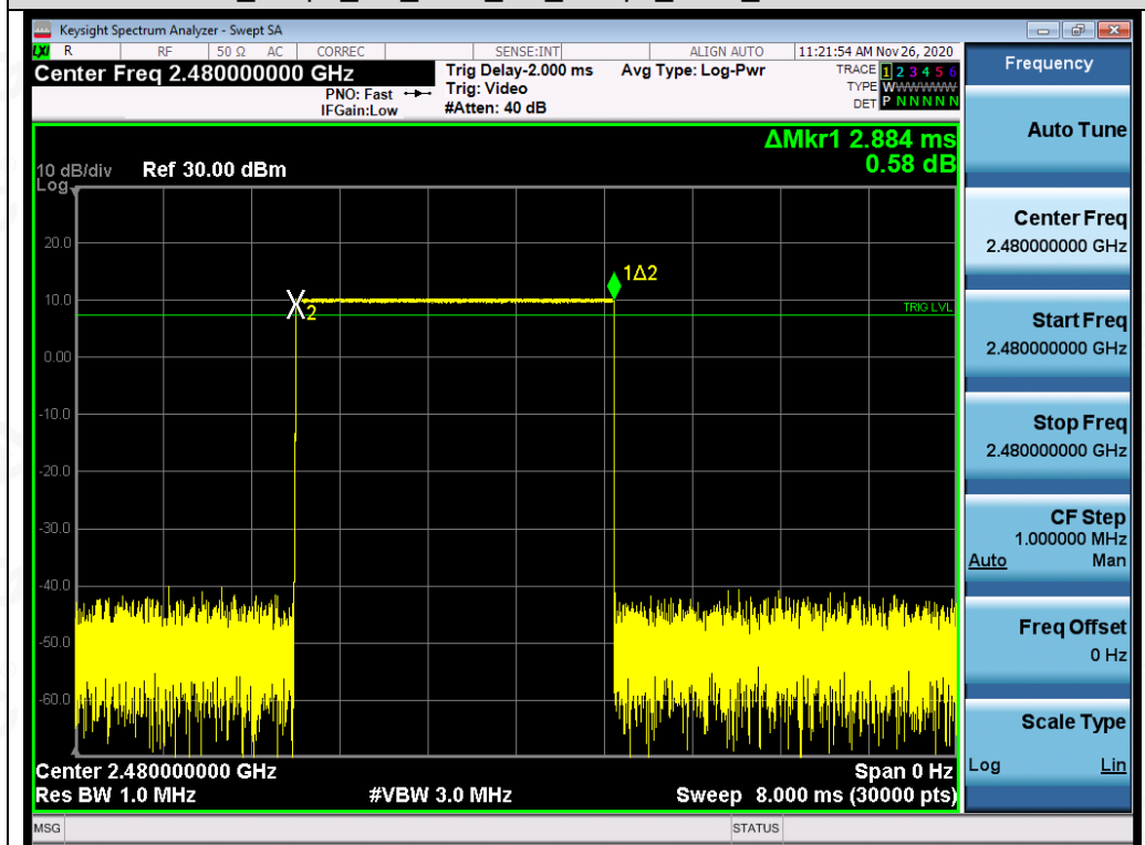
Test_Graph_BR_HOP_NA_1Mbps_2480_Time per Burst
