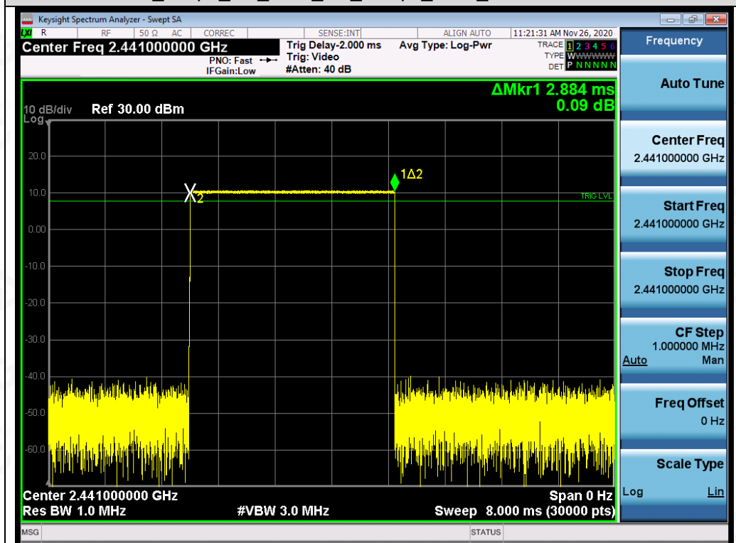
Test_Graph_BR_HOP_NA_1Mbps_2441_Time per Burst
