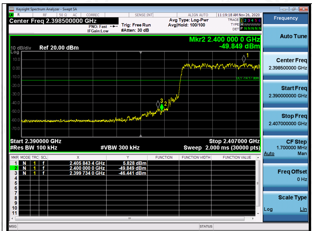
Test_Graph_EDR_HOP_NA_2Mbps_Lower Band Edge Emissions
