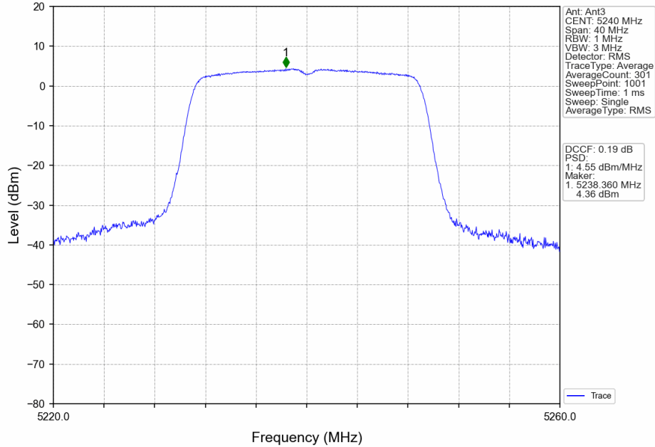
802.11n(HT20)_HCH_5240MHz_MIMO_NTNV
