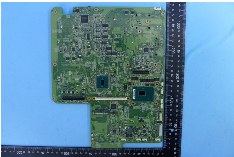
(17) EUT Photo
