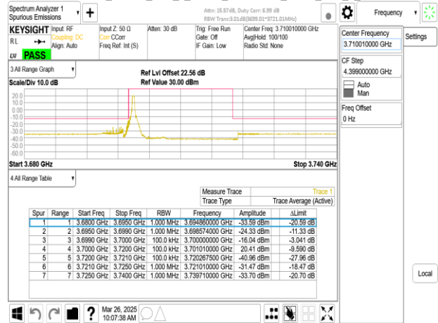
Band77-Part27_20MHz_DFT_s_OFDM_SCS30kHz_BPSK_RB1_50_CH647334
