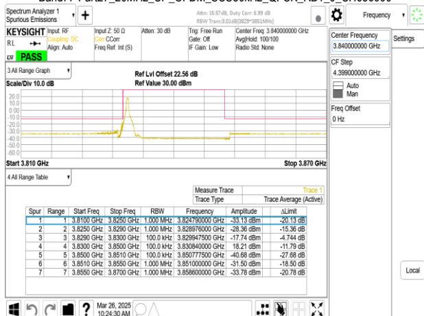
Band77-Part27_20MHz_CP_OFDM_SCS30kHz_QPSK_RB1_50_CH656000
