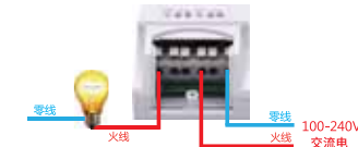
4.2 控制单火线开关正确接线方法 (比如灯具开关)。
