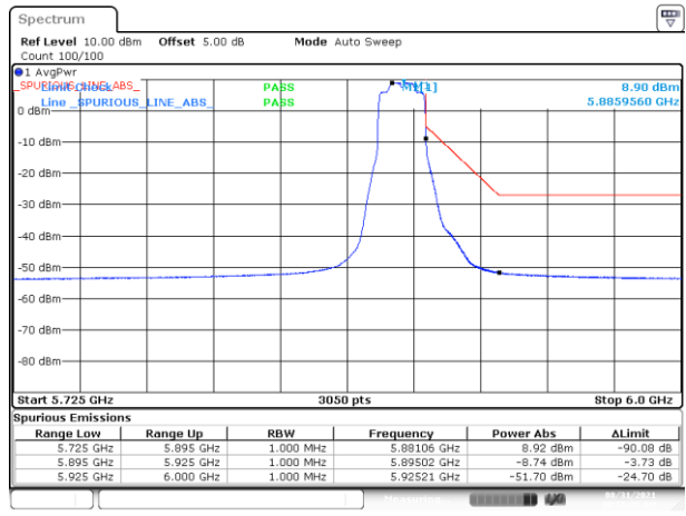
BE-NR-HIGH, MIMO-A, 802.11ax20-MCS0, Ch177
