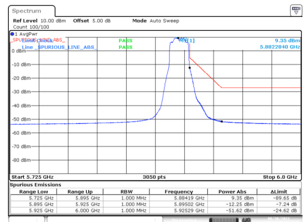
BE-NR-HIGH, MIMO-A, 802.11n20-HT0, Ch177
