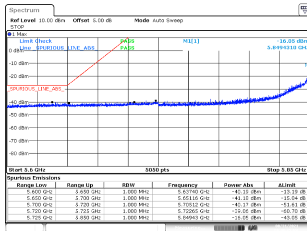
BE-NR-LOW, MIMO-A, 802.11n40-HT0, Ch175
