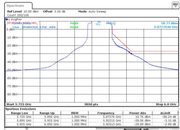
BE-NR-HIGH, SISO-A, 802.11ax40-MCS0, Ch175
