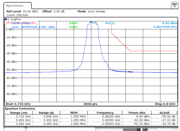
BE-NR-HIGH, MIMO-A, 802.11n20-HT0, Ch173
