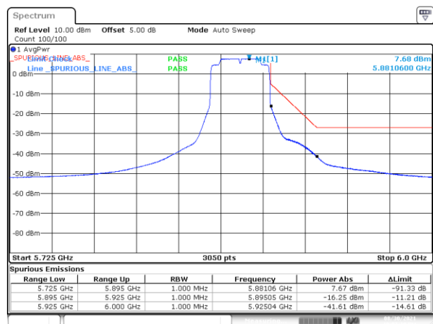
BE-NR-HIGH, MIMO-A, 802.11ax40-MCS0, Ch175
