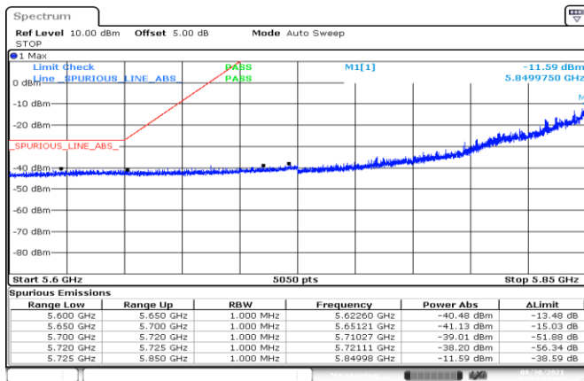
BE-NR-LOW, SISO-A, 802.11ax40-MCS0, Ch175
