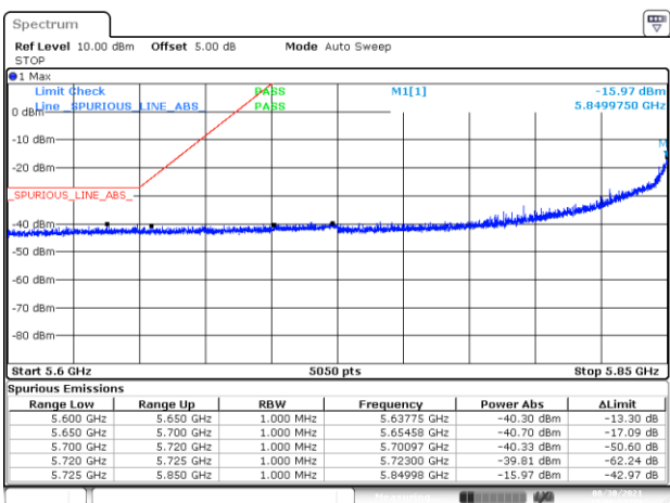
BE-NR-LOW, MIMO-A, 802.11ax40-MCS0, Ch175
