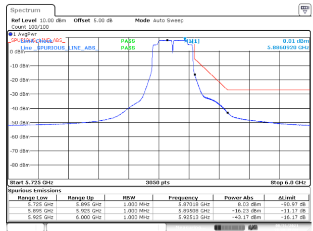
BE-NR-HIGH, MIMO-A, 802.11n40-HT0, Ch175
