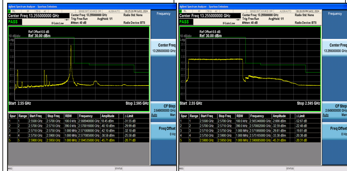
Band7_20MHz_QPSK_21350_1RB#99
