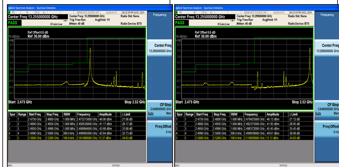
Band7_20MHz_QPSK_21350_1RB#99
