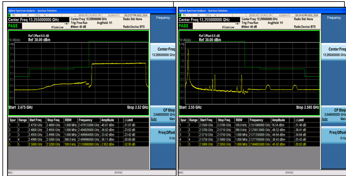
Band7_20MHz_QPSK_20850_100RB#0
