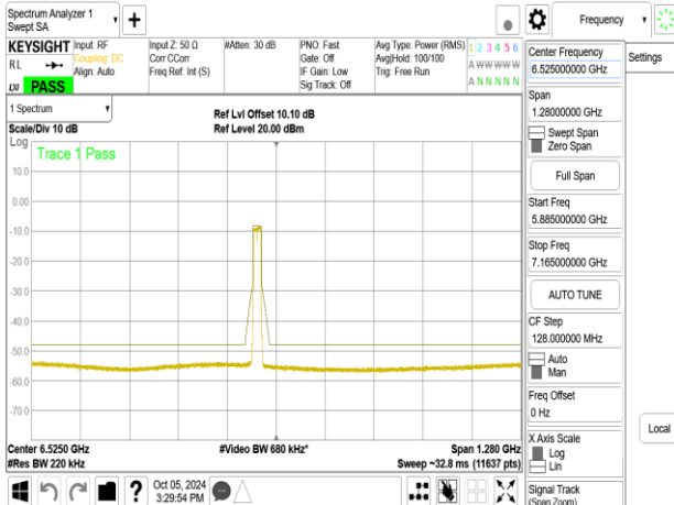
802.11be_20MHz_Chain1_6515MHz
