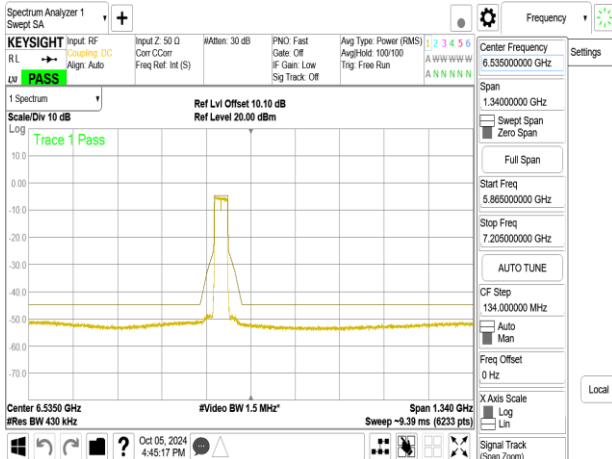
802.11be_40MHz_Chain0_6485MHz
