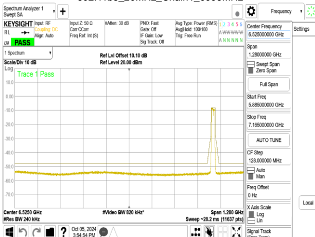
802.11be_20MHz_Chain1_6995MHz
