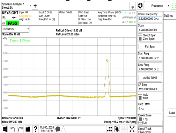
802.11be_20MHz_Chain1_6895MHz
