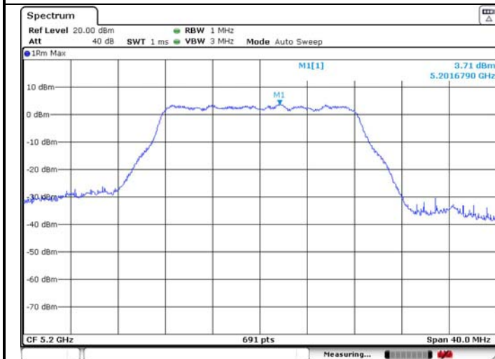
ANT 1
