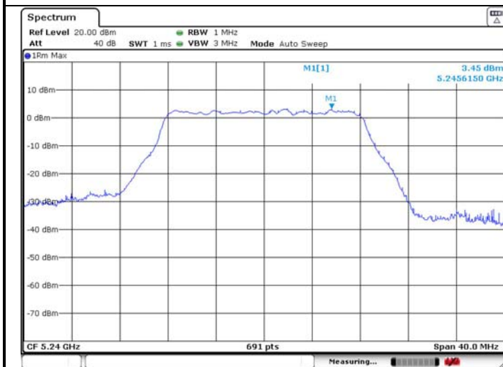
ANT 1
