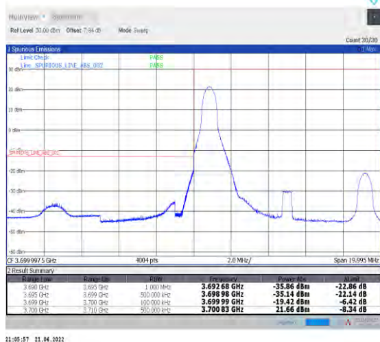
1-N78-3700-3800--30-10-L-4-CP-QPSK-Edge_1RB_L eft-1@0-Ant0-PASS-see graph
