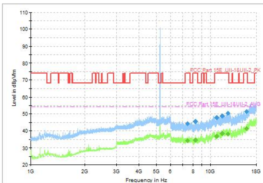
Fig. 56 Transmitter Spurious Emission (802.11ax-HE20(RU26), CH48 5240MHz, 1GHz-18GHz)
