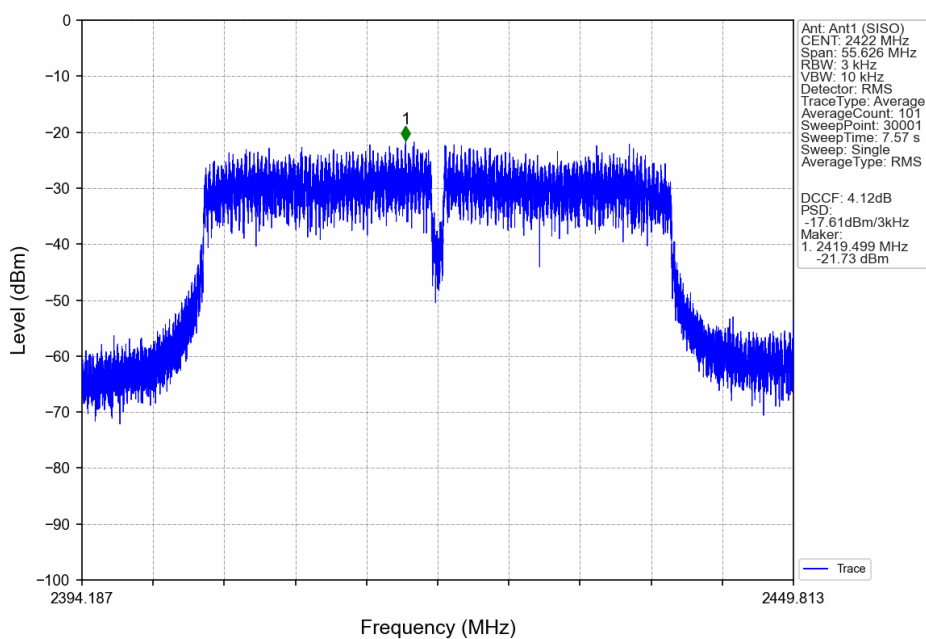
802.11n(HT40)_LCH_2422MHz_Ant1 (SISO)_NTNV
