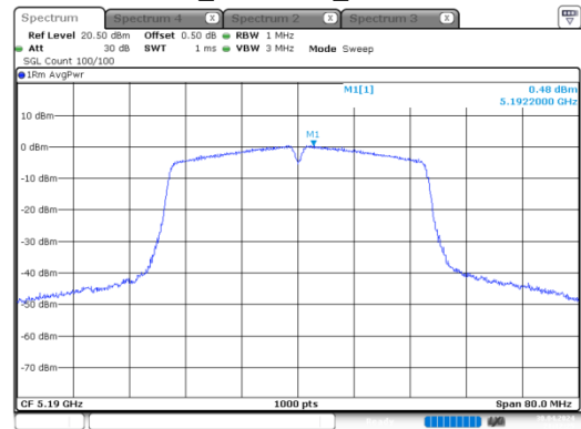
n40_5190MHz_Chain 1
