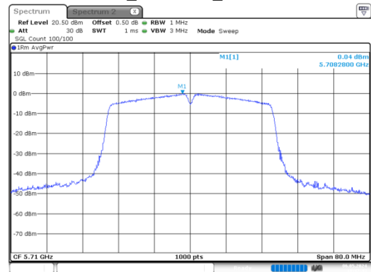
n40_5710MHz_Chain 1
