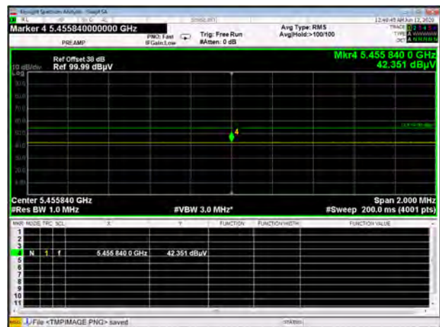
Band III 11ac20 CH100 AV
