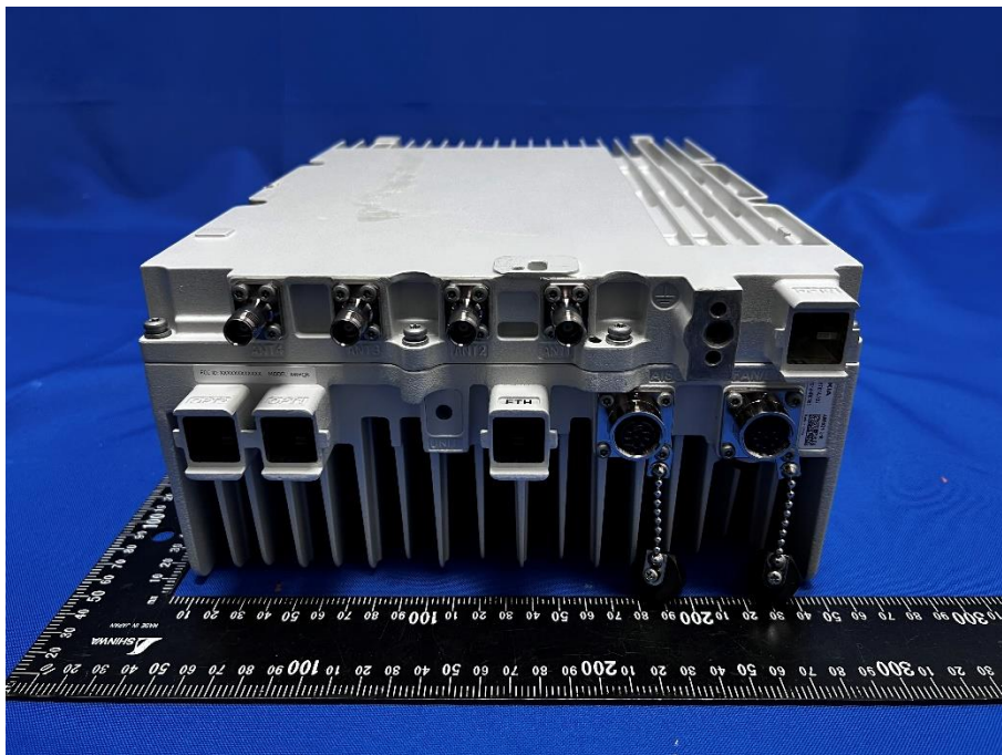
(3) EUT Photo
