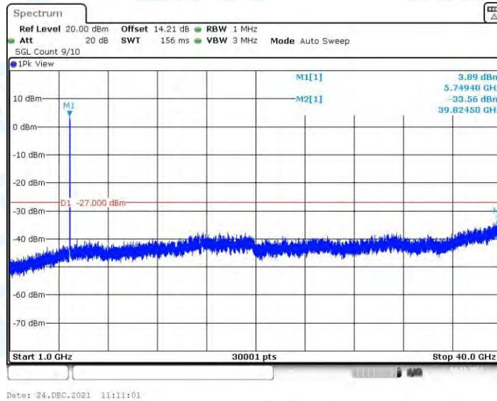
11N40MIMO_Ant3_5755_1000~40000
