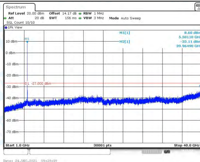
11N20MIMO_Ant2_5500_1000~40000
