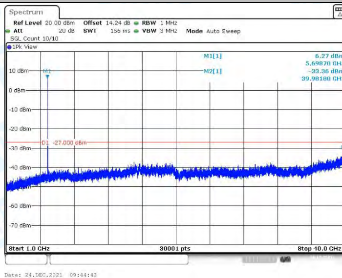
11N20MIMO_Ant2_5700_1000~40000
