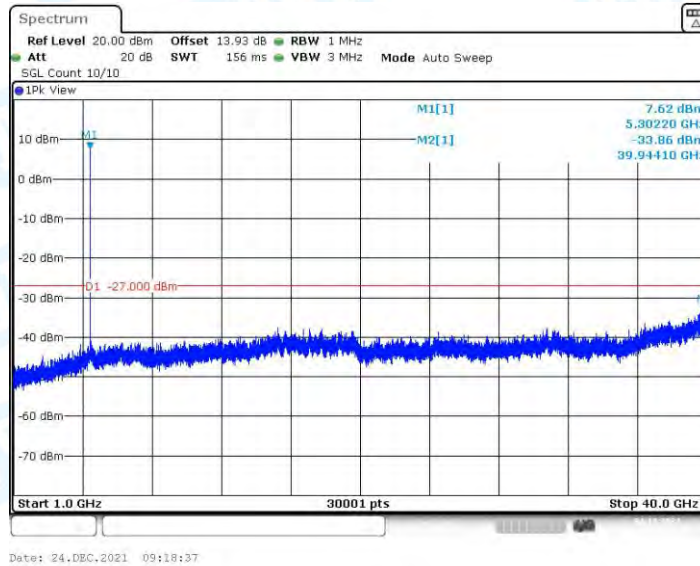
11N20MIMO_Ant3_5300_1000~40000
