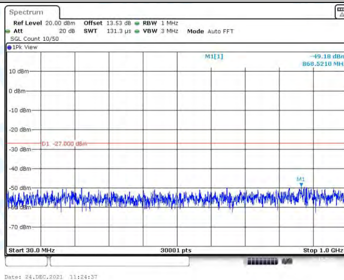
11AC20MIMO_Ant1_5180_30~1000
