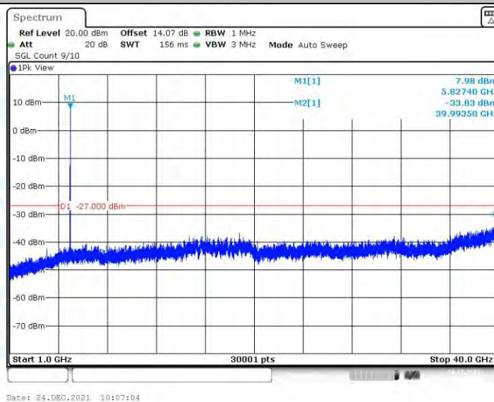
11N20MIMO_Ant2_5825_1000~40000
