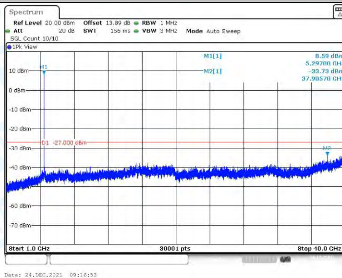
11N20MIMO_Ant2_5300_1000~40000
