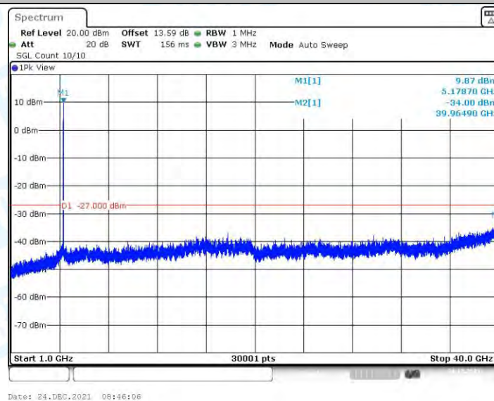
11N20MIMO_Ant2_5180_1000~40000
