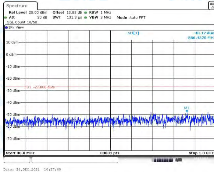
11N40MIMO_Ant3_5270_30~1000
