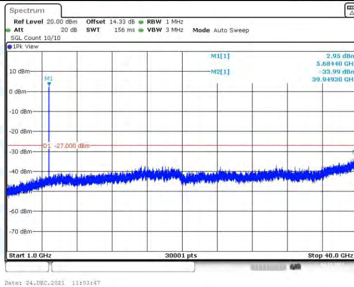
11N40MIMO_Ant3_5670_1000~40000
