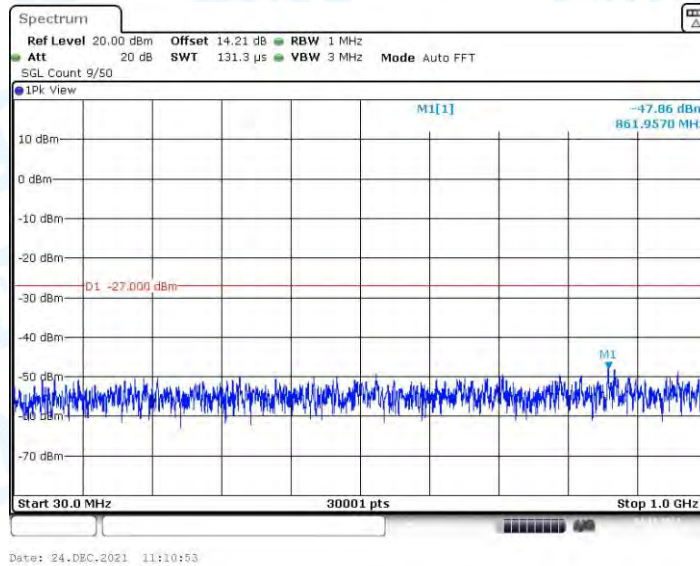
11N40MIMO_Ant3_5755_30~1000
