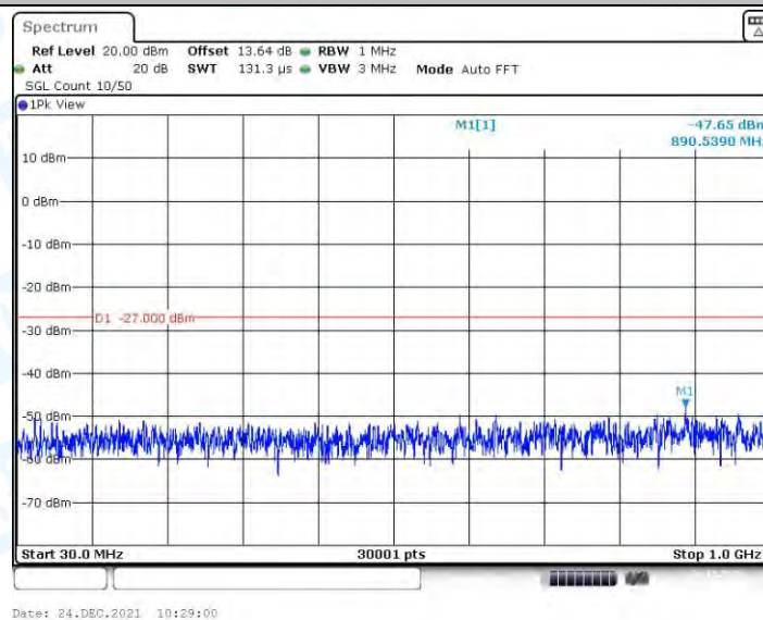
11N40MIMO_Ant1_5310_30~1000
