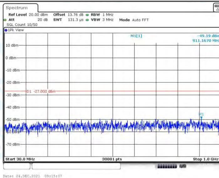
11N20MIMO_Ant1_5300_30~1000
