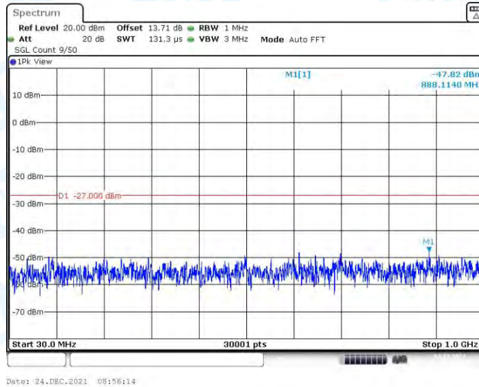
11N20MIMO_Ant3_5220_30~1000
