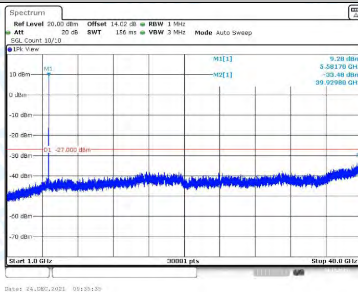
11N20MIMO_Ant2_5580_1000~40000
