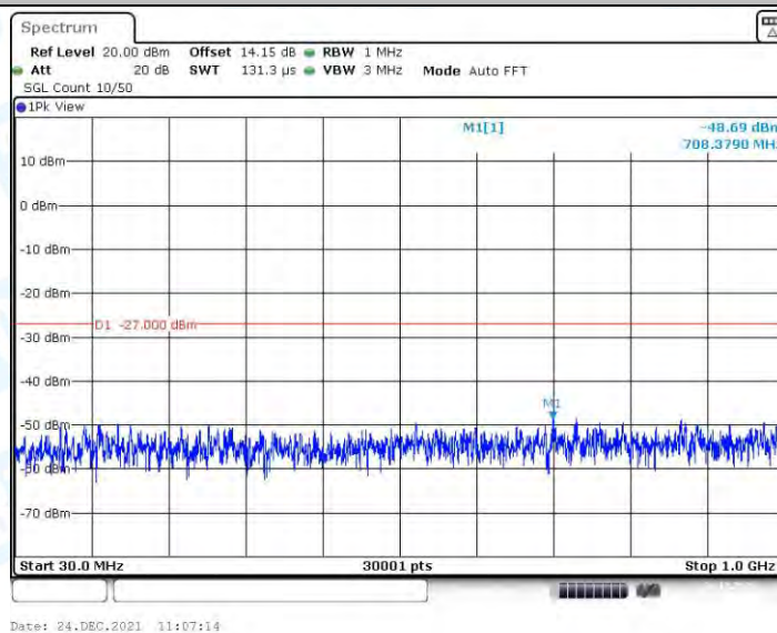
11N40MIMO_Ant1_5755_30~1000
