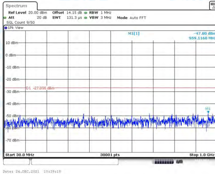
11N40MIMO_Ant3_5510_30~1000
