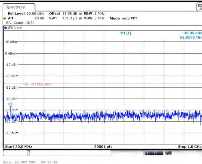
11N20MIMO_Ant1_5580_30~1000
