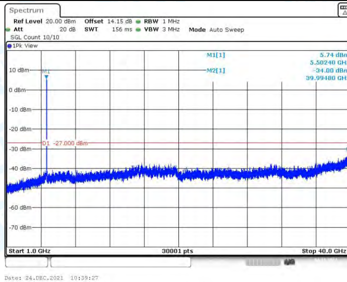
11N40MIMO_Ant3_5510_1000~40000
