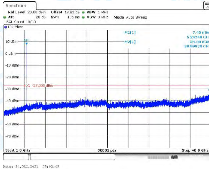
11N20MIMO_Ant3_5240_1000~40000
