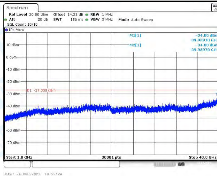
11N40MIMO_Ant2_5670_1000~40000
