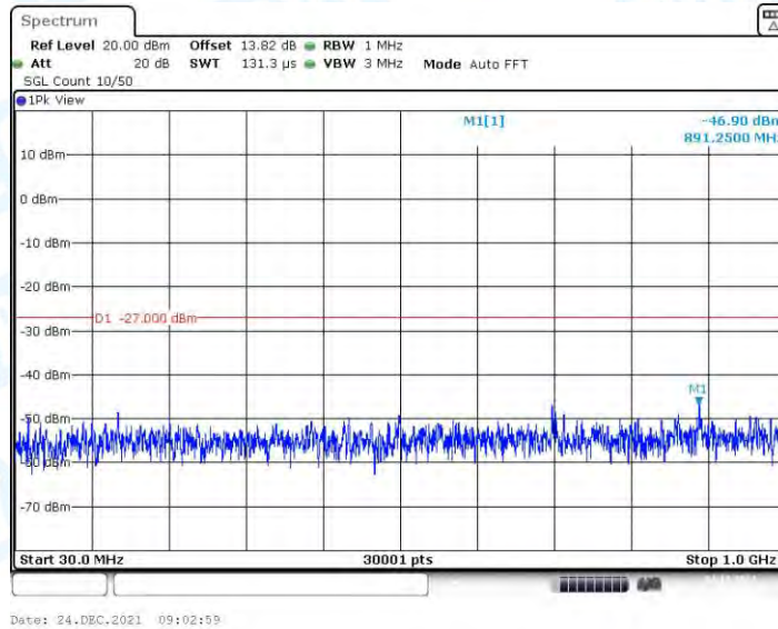
11N20MIMO_Ant3_5240_30~1000
