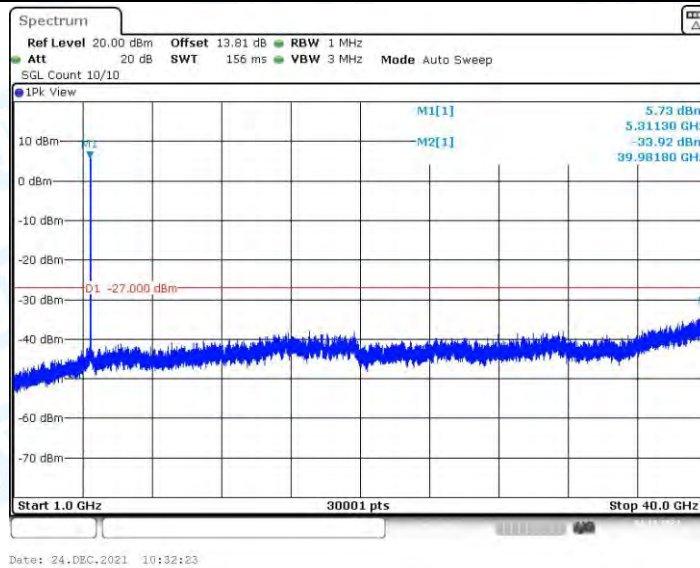
11N40MIMO_Ant3_5310_1000~40000
