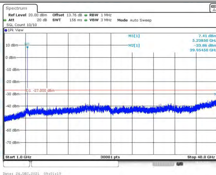
11N20MIMO_Ant2_5240_1000~40000
