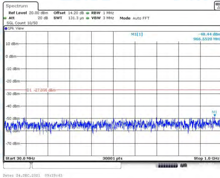
11N20MIMO_Ant3_5500_30~1000
