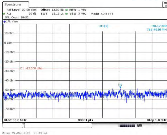
11N40MIMO_Ant3_5230_30~1000
