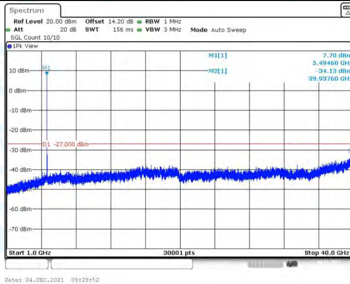
11N20MIMO_Ant3_5500_1000~40000
