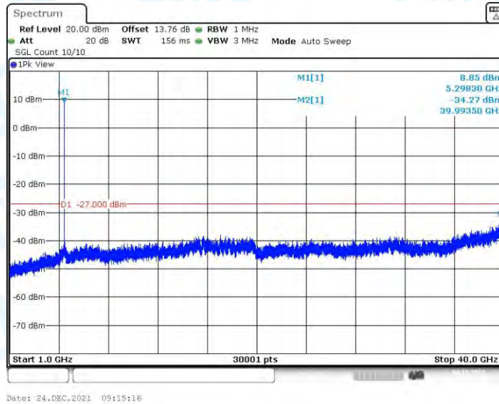
11N20MIMO_Ant1_5300_1000~40000
