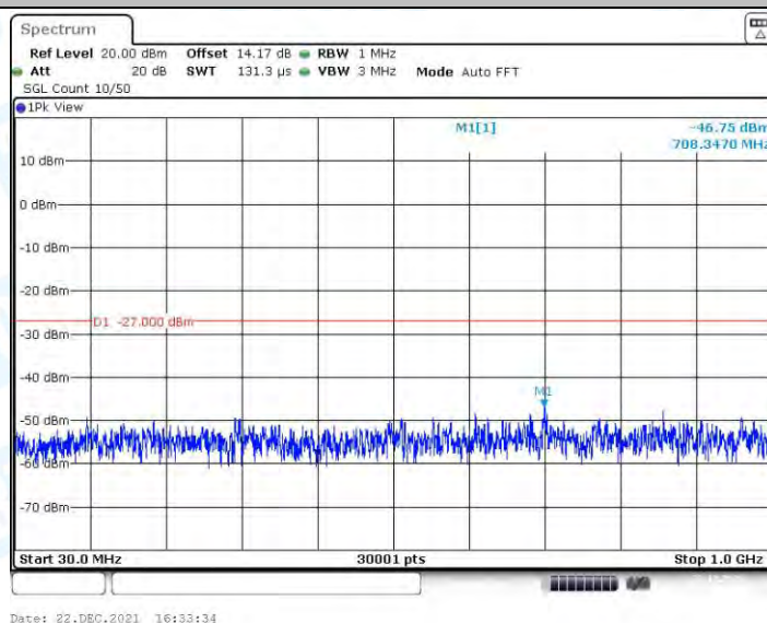
11A_Ant2_5500_30~1000
