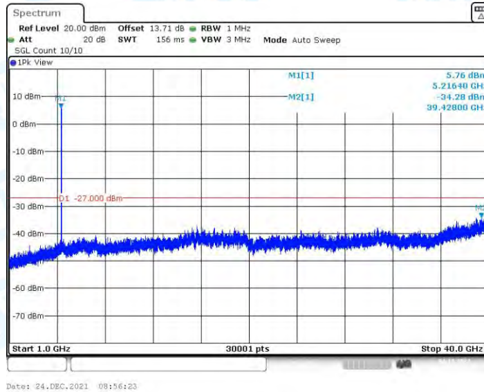
11N20MIMO_Ant3_5220_1000~40000
