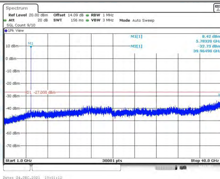
11N20MIMO_Ant3_5785_1000~40000
