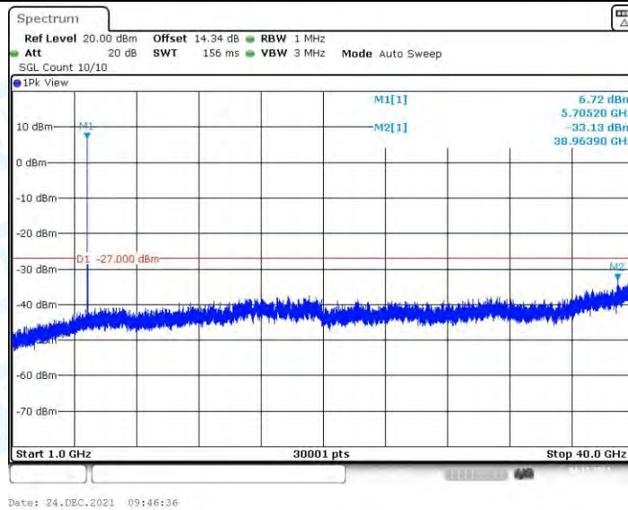
11N20MIMO_Ant3_5700_1000~40000
