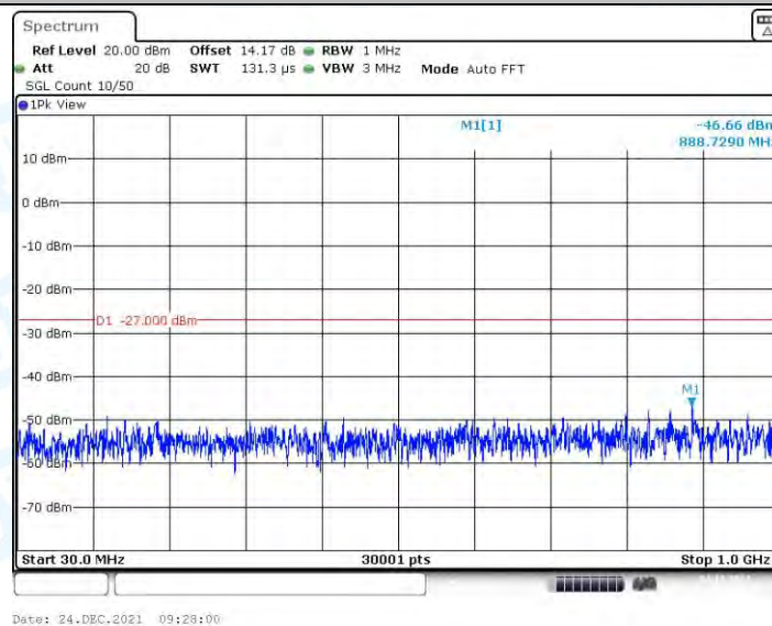
11N20MIMO_Ant2_5500_30~1000
