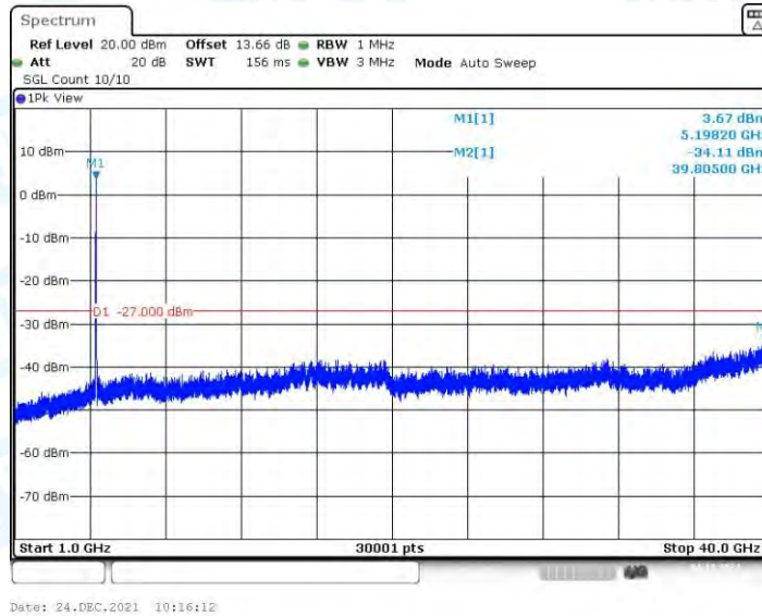
11N40MIMO_Ant3_5190_1000~40000
