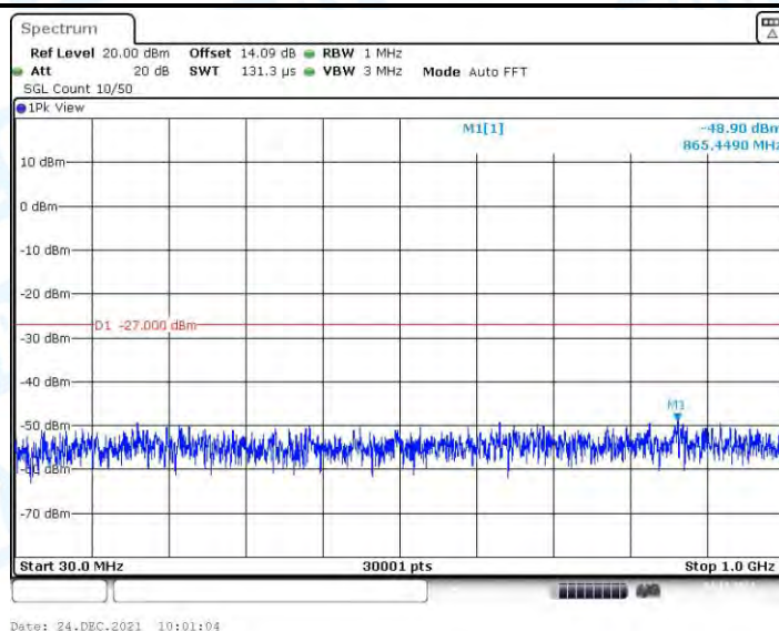
11N20MIMO_Ant3_5785_30~1000
