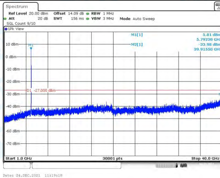
11N40MIMO_Ant3_5795_1000~40000
