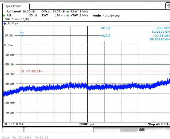
11N20MIMO_Ant2_5320_1000~40000
