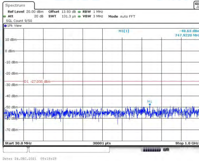
11N20MIMO_Ant3_5300_30~1000
