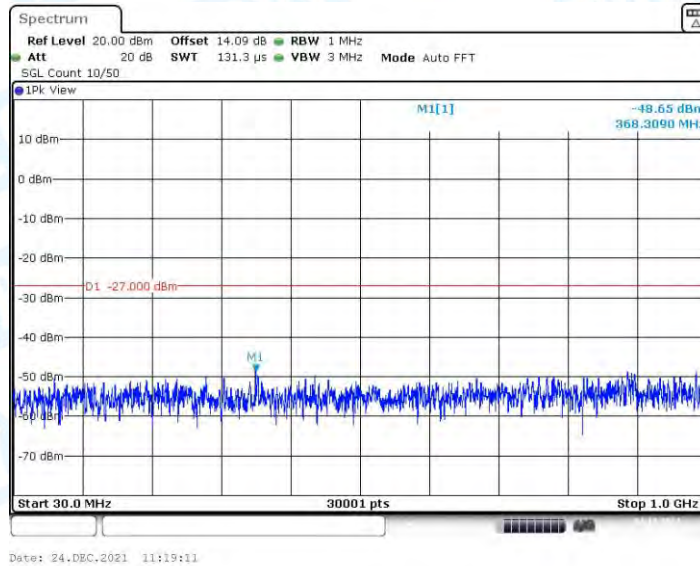
11N40MIMO_Ant3_5795_30~1000
