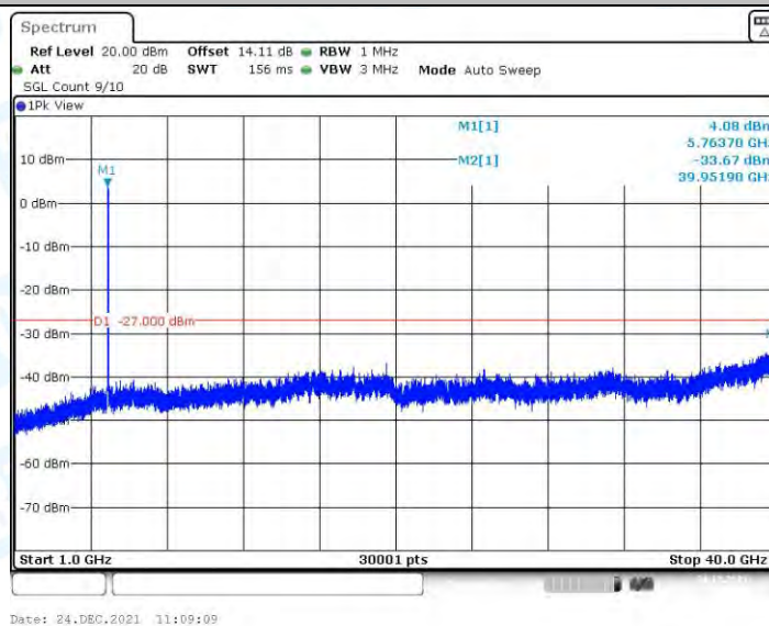
11N40MIMO_Ant2_5755_1000~40000
