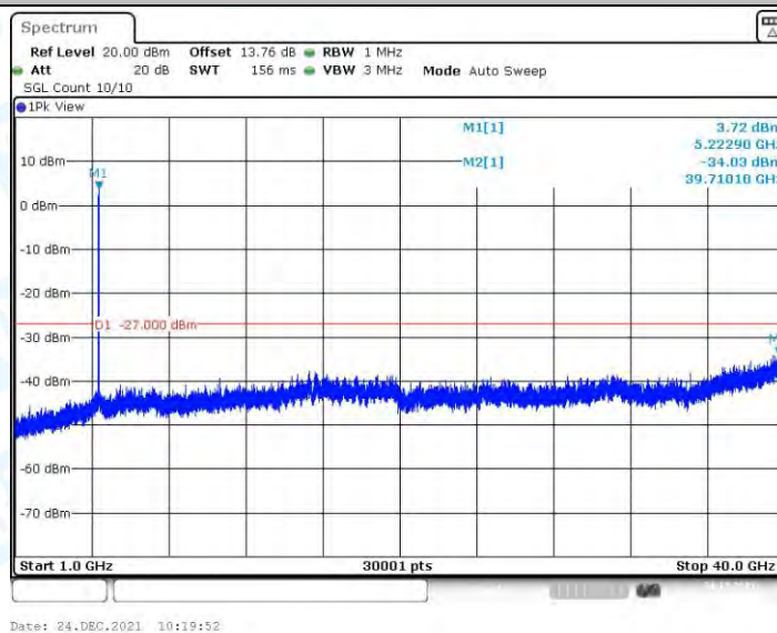
11N40MIMO_Ant2_5230_1000~40000
