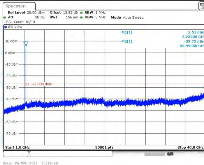
11N40MIMO_Ant3_5230_1000~40000
