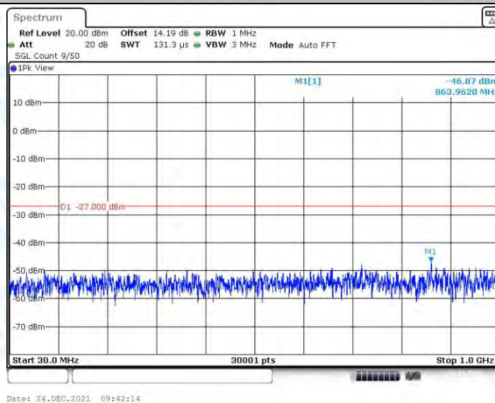
11N20MIMO_Ant1_5700_30~1000
