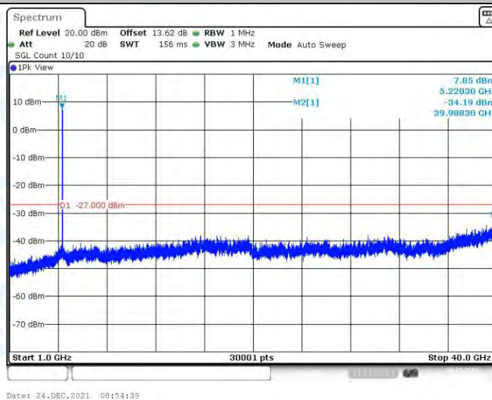
11N20MIMO_Ant2_5220_1000~40000
