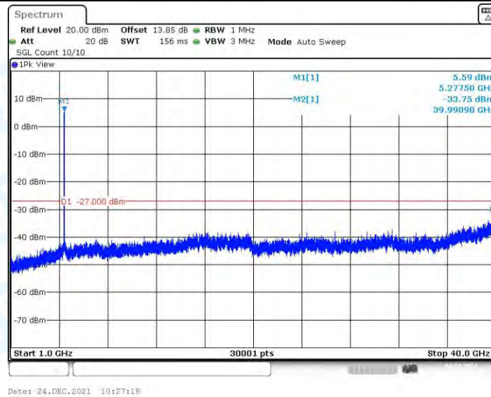
11N40MIMO_Ant3_5270_1000~40000
