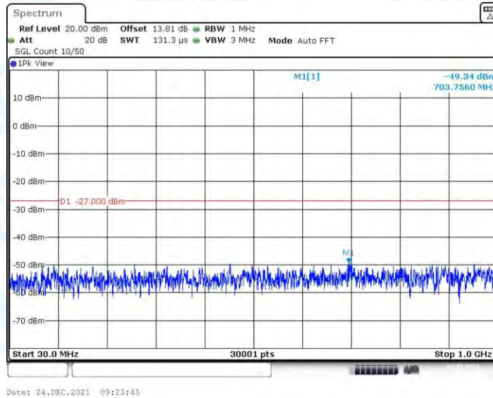
11N20MIMO_Ant3_5320_30~1000
