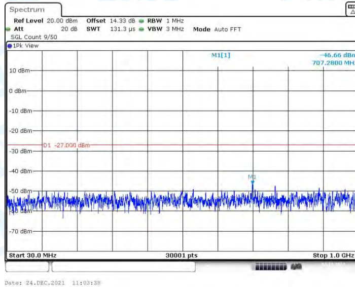
11N40MIMO_Ant3_5670_30~1000
