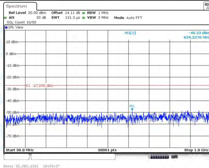
11A_Ant3_5580_30~1000
