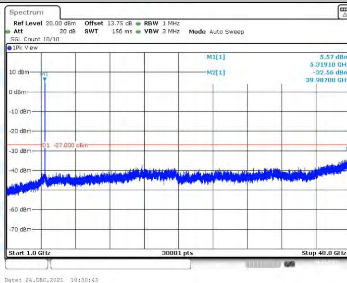
11N40MIMO_Ant2_5310_1000~40000
