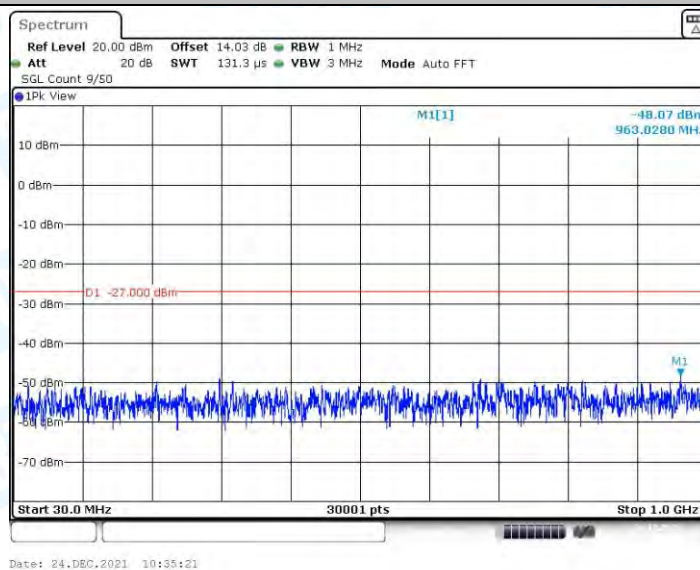
11N40MIMO_Ant1_5510_30~1000
