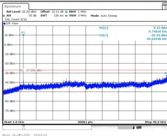
11N20MIMO_Ant2_5745_1000~40000
