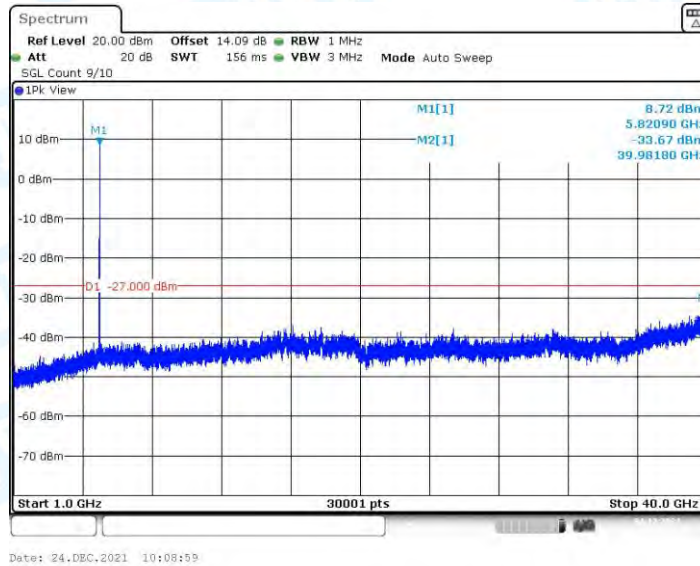
11N20MIMO_Ant3_5825_1000~40000
