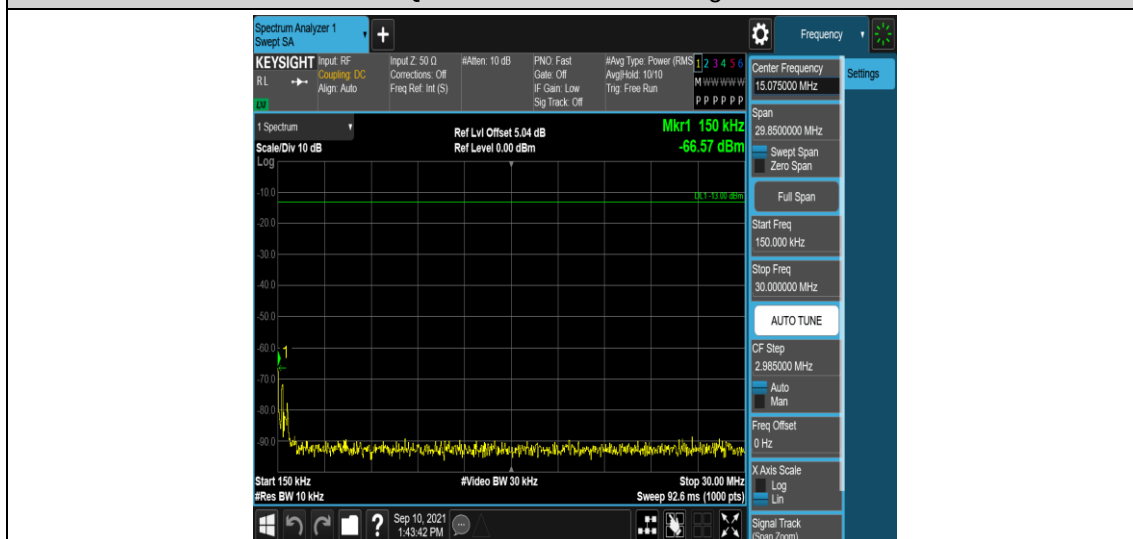
Band26-1.4MHz-QPSK-26783-1RB#0-Range2:0.15~30MHz
