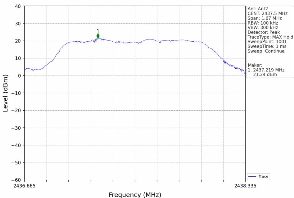
1.4M_MCH_2437.5MHz_Ant2_NTNV
