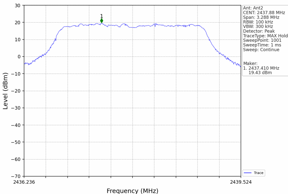
3M_MCH_2437.88MHz_Ant2_NTNV
