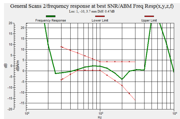
WCDMA1900
