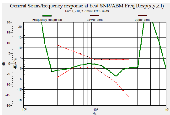
WCDMA850
