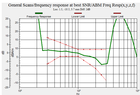
CDMA800 (BC0)
