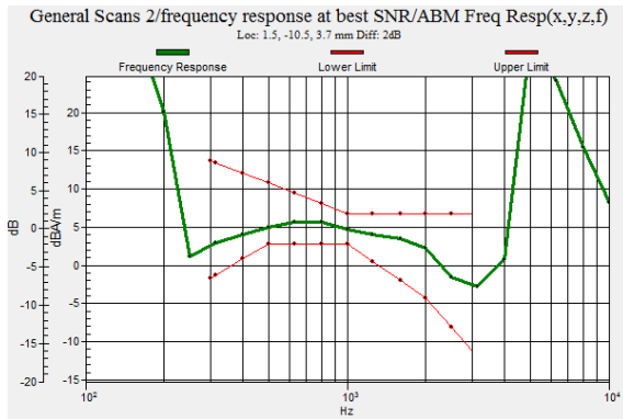
GSM850
