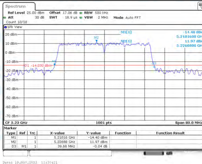
11N40-CDD_Ant3_5230
