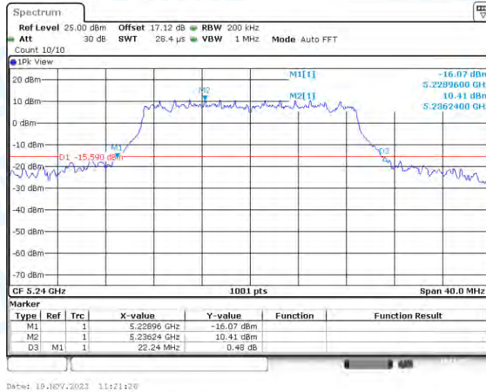
11N20-CDD_Ant4_5240
