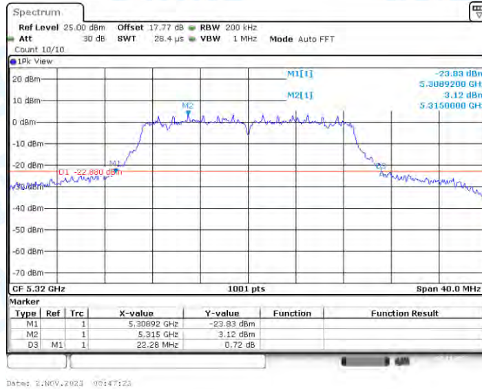
11N20-CDD_Ant4_5320
