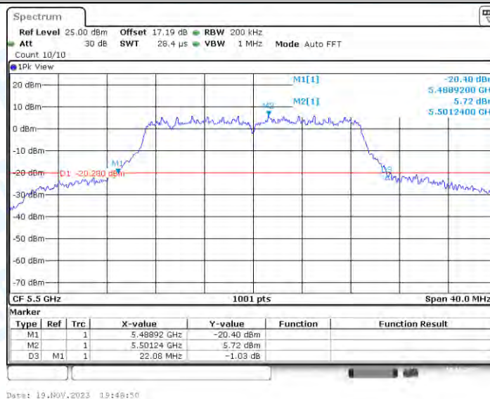
11AC20-CDD_Ant2_5500
