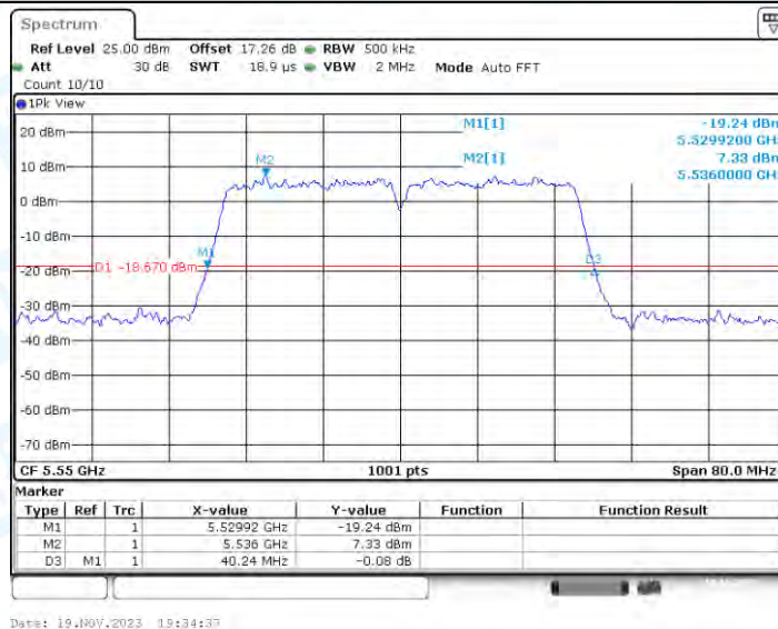
11N40-CDD_Ant2_5550
