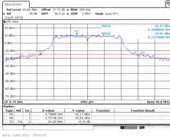
11A_Ant3_5720
