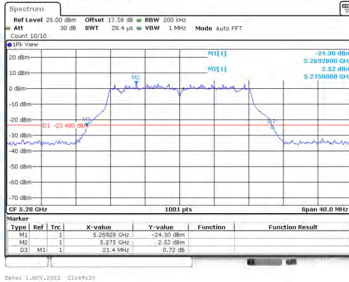
11A-CDD_Ant3_5280
