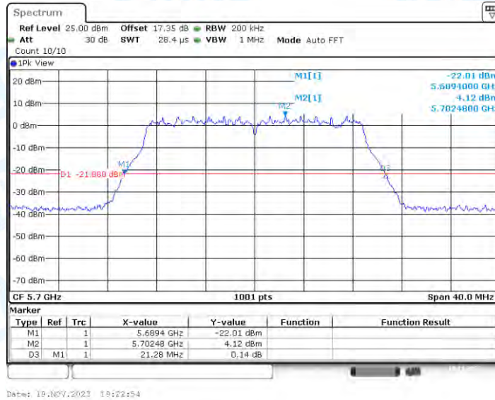
11N20-CDD_Ant4_5700
