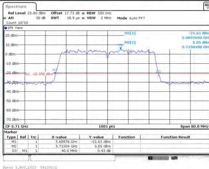
11N40-CDD_Ant3_5710
