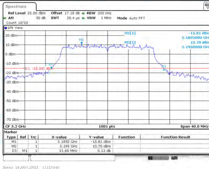
11N20-CDD_Ant4_5200
