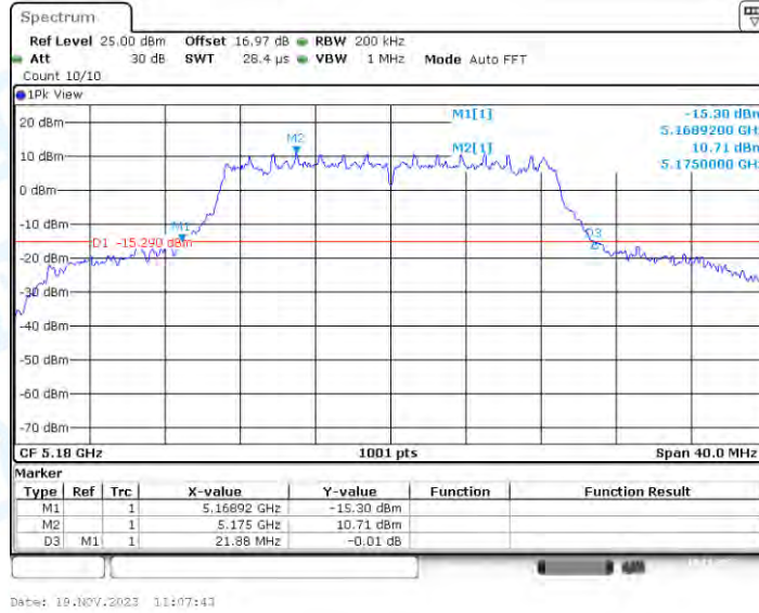
11N20-CDD_Ant3_5180
