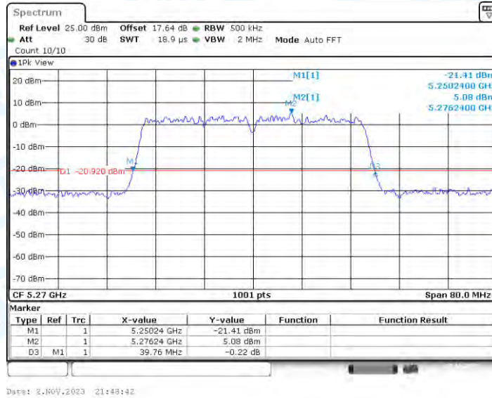
11N40-CDD_Ant4_5270
