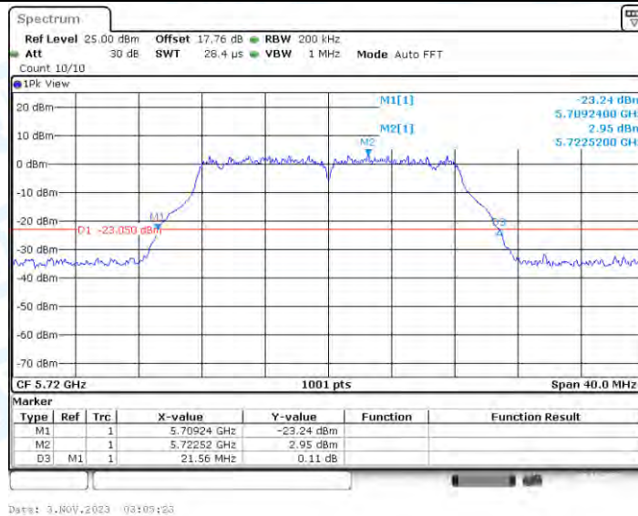
11A-CDD_Ant2_5720
