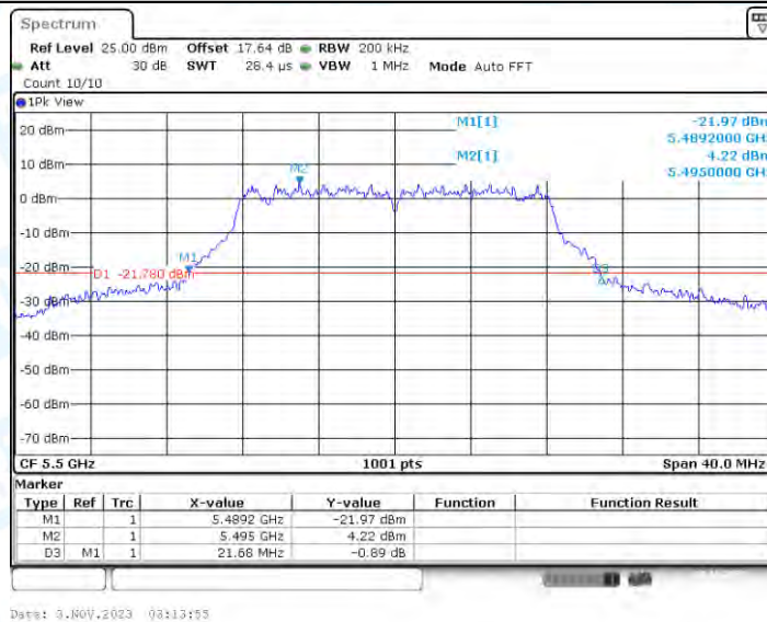
11A-CDD_Ant3_5500
