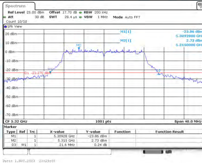
11A-CDD_Ant3_5320
