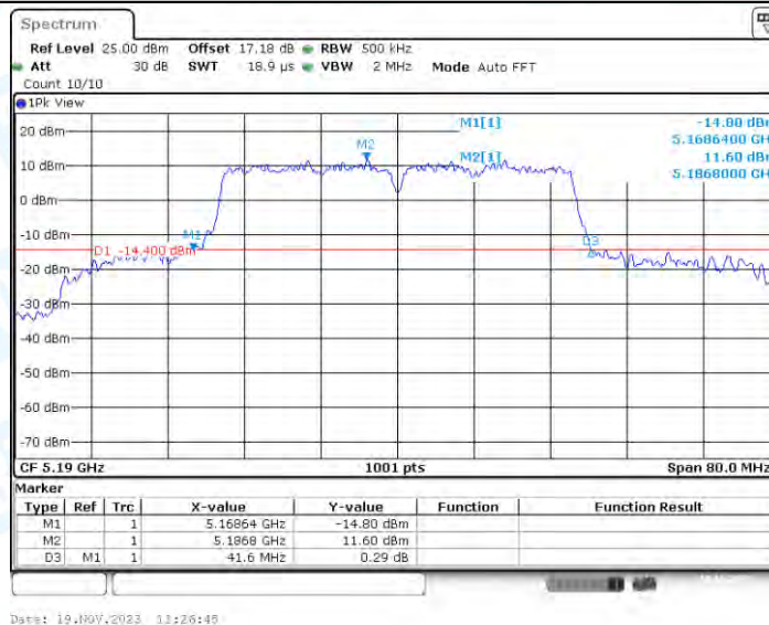
11N40-CDD_Ant4_5190
