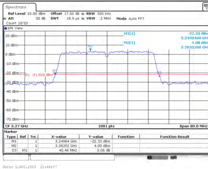
11N40-CDD_Ant2_5270
