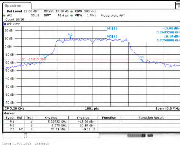
11A_Ant3_5280
