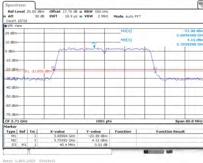
11N40-CDD_Ant2_5710
