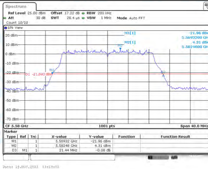
11N20-CDD_Ant4_5580
