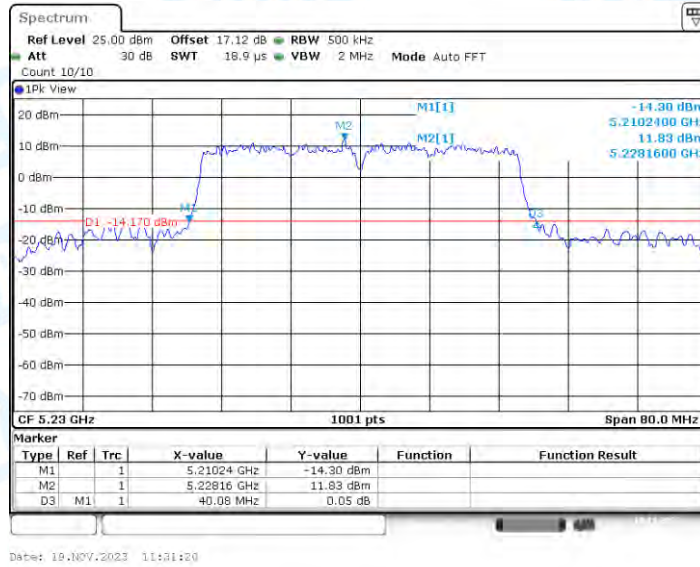
11N40-CDD_Ant4_5230
