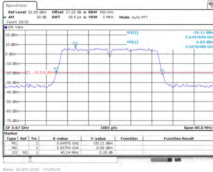
11N40-CDD_Ant2_5670
