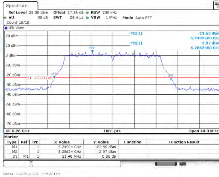
11N20-CDD_Ant3_5260
