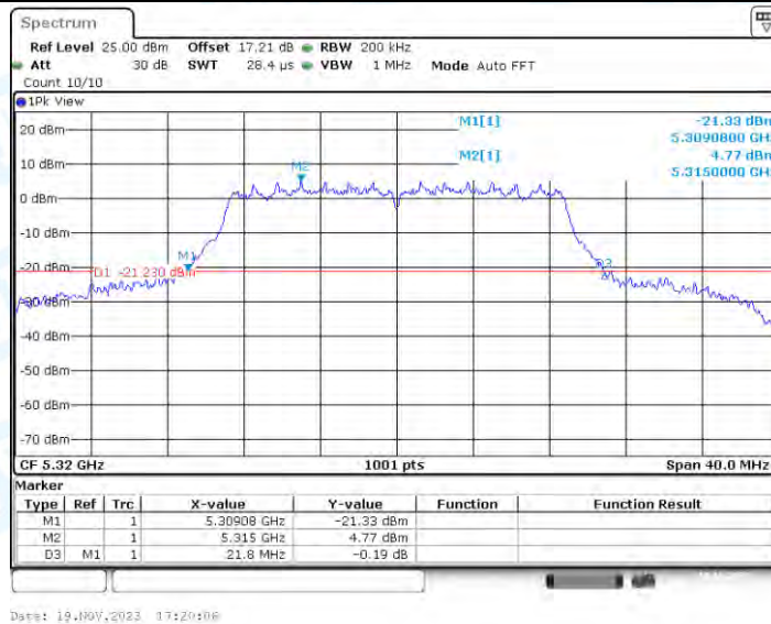
11AC20-CDD_Ant2_5320
