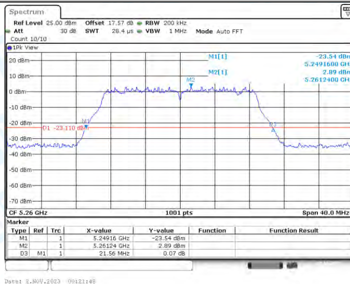
11N20-CDD_Ant2_5260
