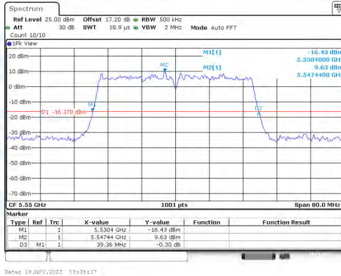
11N40-CDD_Ant3_5550
