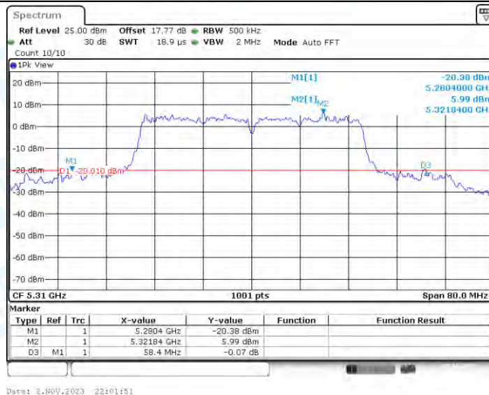
11N40-CDD_Ant4_5310
