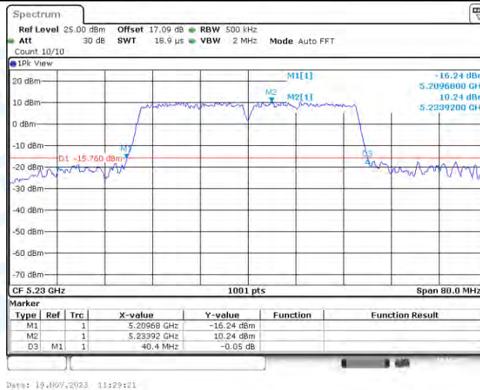
11N40-CDD_Ant2_5230
