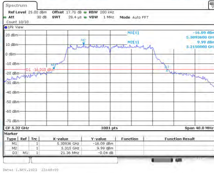
11A_Ant3_5320
