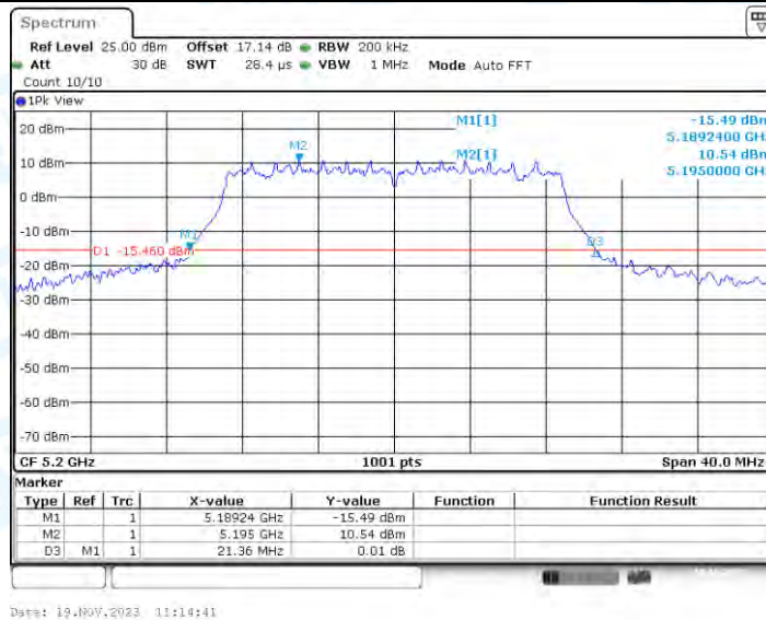
11N20-CDD_Ant3_5200
