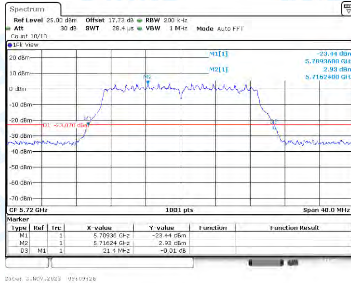
11N20-CDD_Ant3_5720
