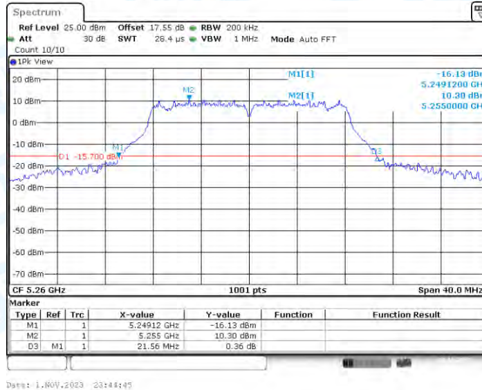
11A_Ant3_5260
