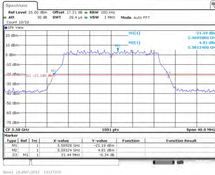
11N20-CDD_Ant3_5580
