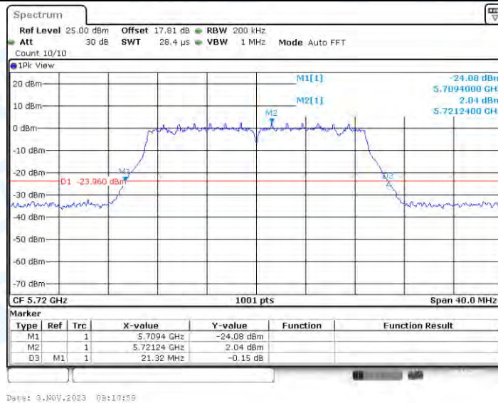
11N20-CDD_Ant4_5720
