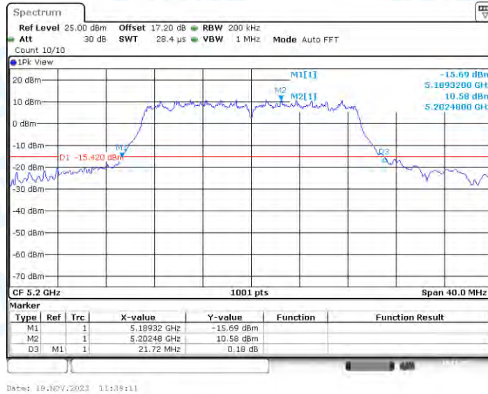
11AC20-CDD_Ant2_5200
