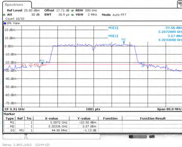
11N40-CDD_Ant2_5310
