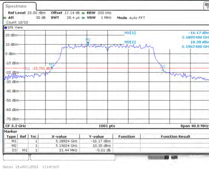
11AC20-CDD_Ant3_5200
