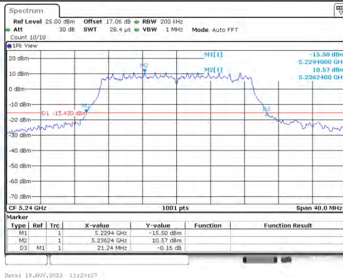
11N20-CDD_Ant3_5240
