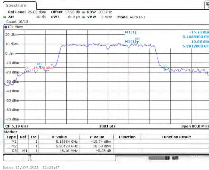
11N40-CDD_Ant2_5190
