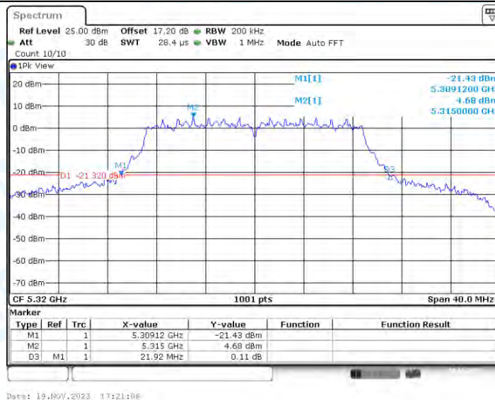
11AC20-CDD_Ant3_5320
