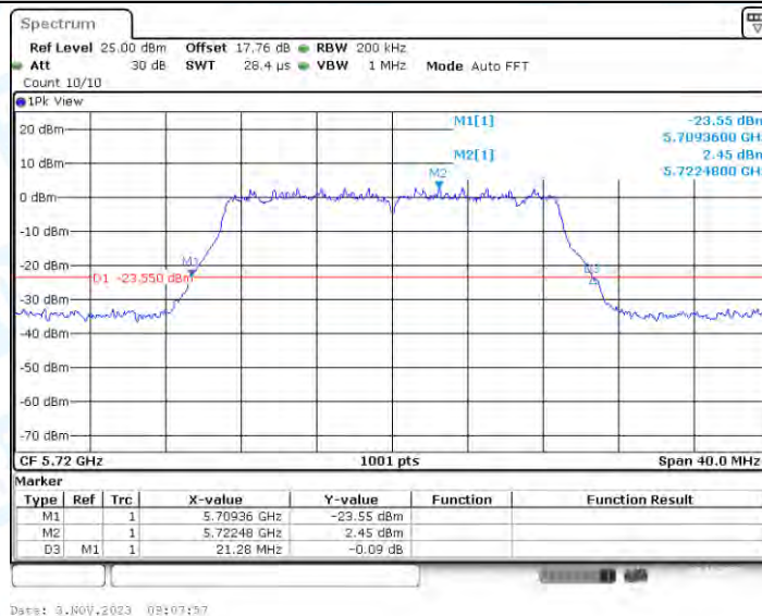
11N20-CDD_Ant2_5720
