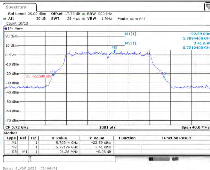
11A-CDD_Ant3_5720
