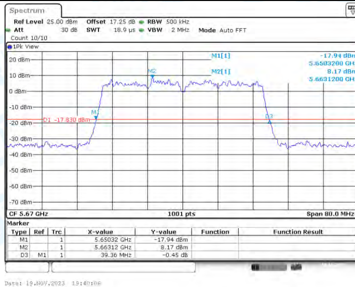
11N40-CDD_Ant3_5670
