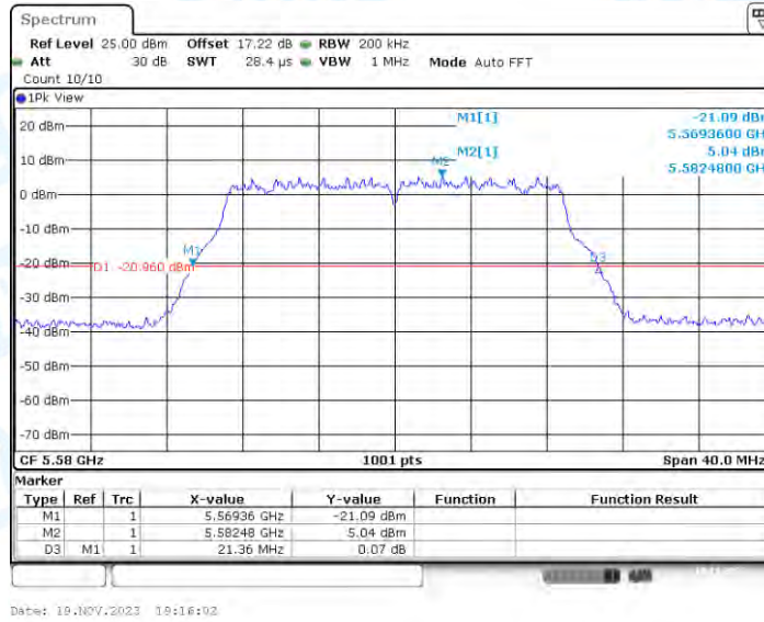
11N20-CDD_Ant2_5580
