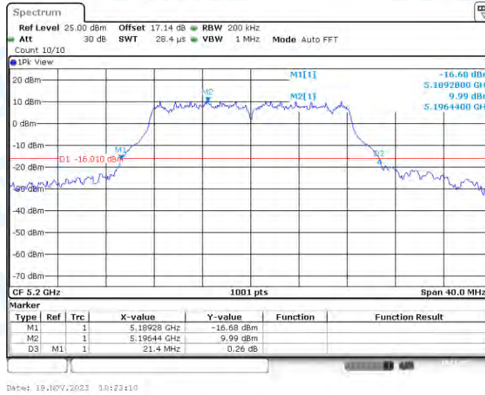
11A-CDD_Ant3_5200
