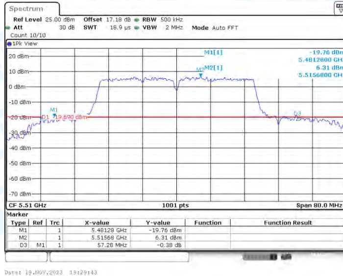
11N40-CDD_Ant2_5510
