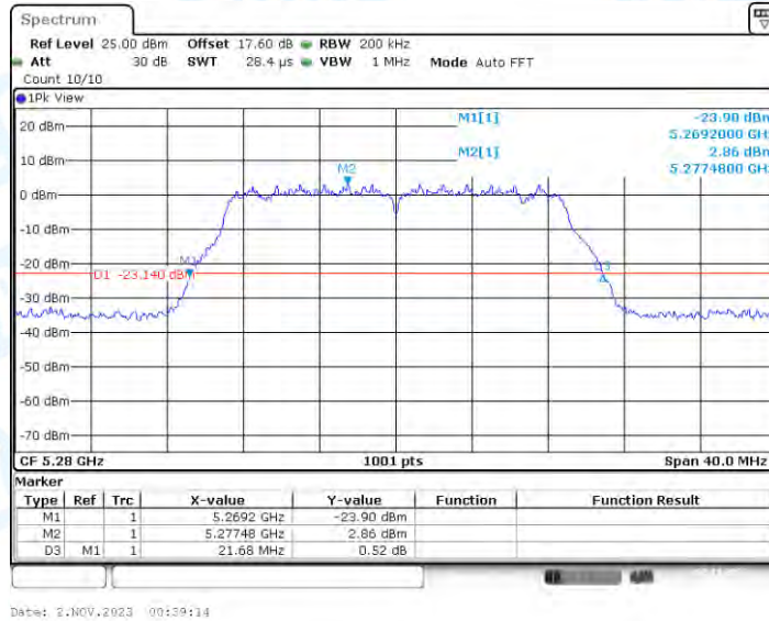
11N20-CDD_Ant2_5280
