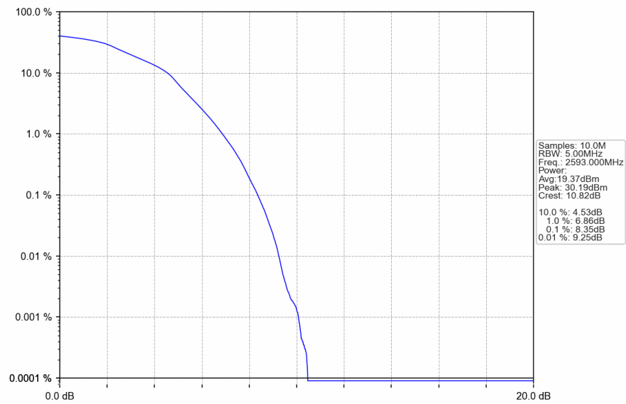
Band41_5MHz_16QAM_MCH_2593.000MHz_RB_25_0_NTNV
