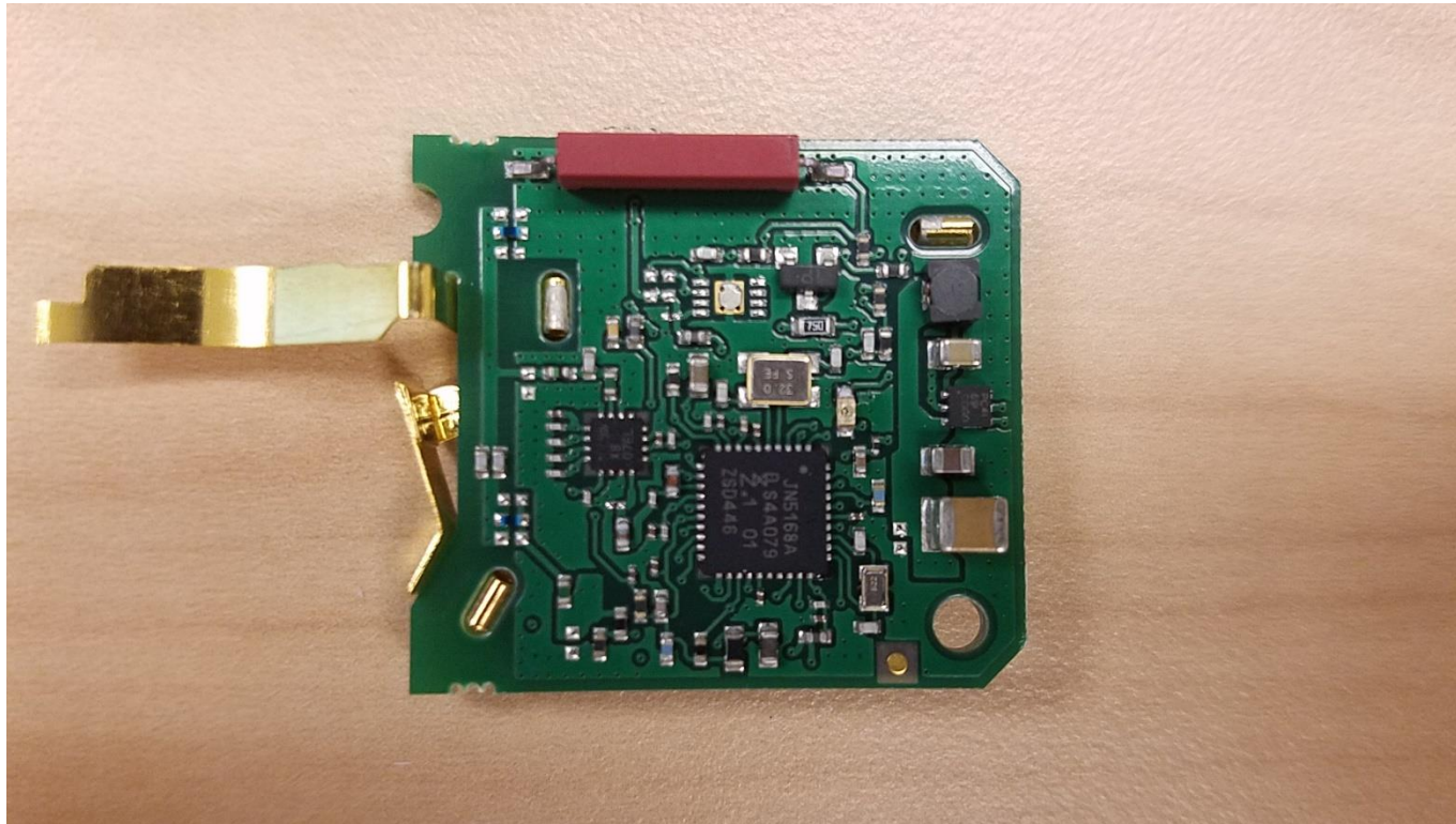
PCB - Bottom
