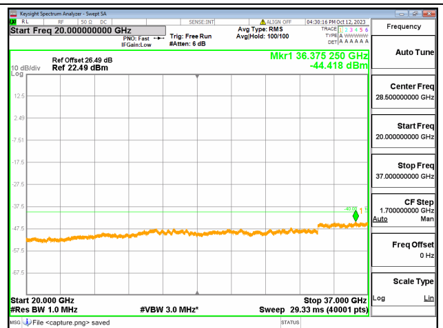
48C-20G-37G / 20+10MHz / QPSK / Mid CH / 1#99-1#0
