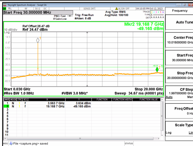
48C-30M-20G / 20+15MHz / QPSK / Low CH / 100#0-75#0
