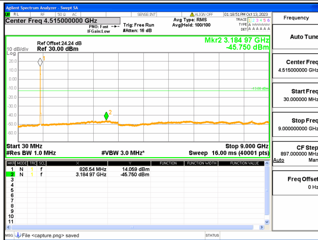
5B / 5+10MHz / QPSK / Low CH / 25#0-50#0
