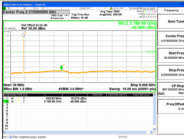
5B / 5+3MHz / QPSK / Mid CH / 25#0-15#0
