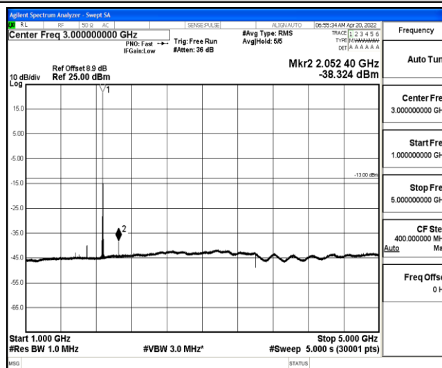
Band25-20MHz-QPSK-26365-1-0-Low-1000-5000--38.32-PASS
