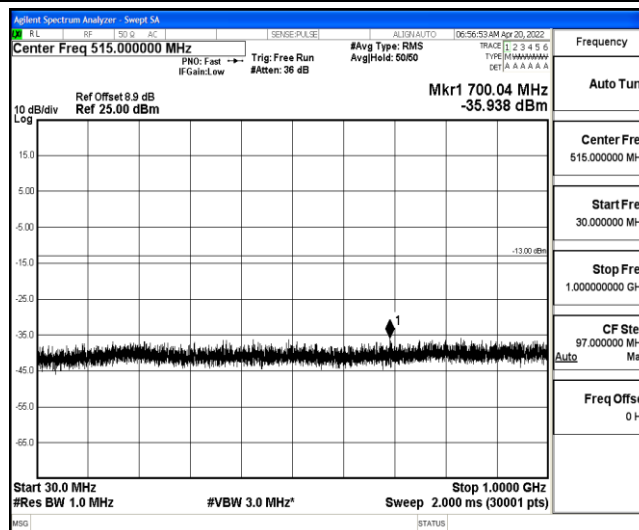
Band25-20MHz-16QAM-26365-1-0-Low-30-1000--35.94-PASS
