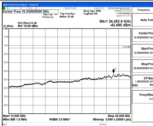
Band25-20MHz-QPSK-26365-1-0-Low-12000-26500--42.5-PASS
