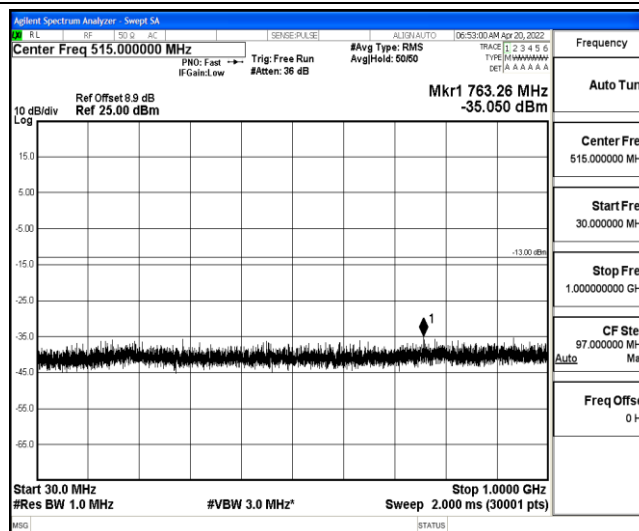
Band25-20MHz-16QAM-26140-1-0-Low-30-1000--35.05-PASS
