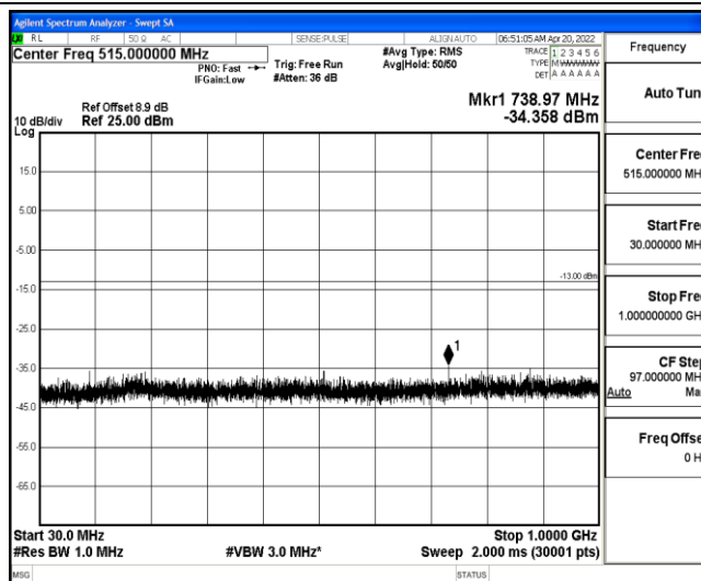
Band25-20MHz-QPSK-26140-1-0-Low-30-1000--34.36-PASS
