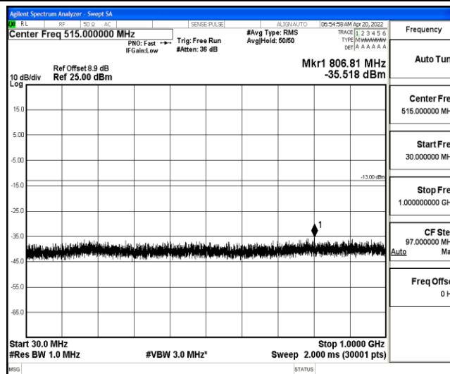
Band25-20MHz-QPSK-26365-1-0-Low-30-1000--35.52-PASS
