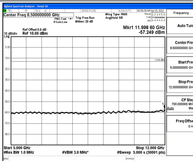
Band25-20MHz-QPSK-26365-1-0-Low-5000-12000--57.25-PASS
