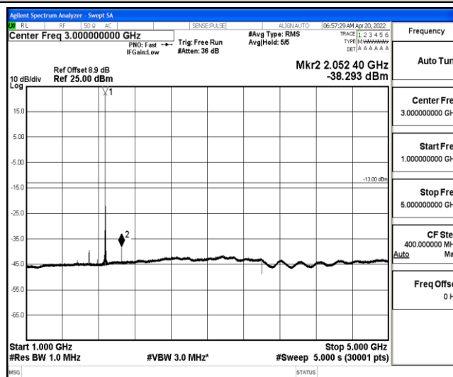
Band25-20MHz-16QAM-26365-1-0-Low-1000-5000--38.29-PASS
