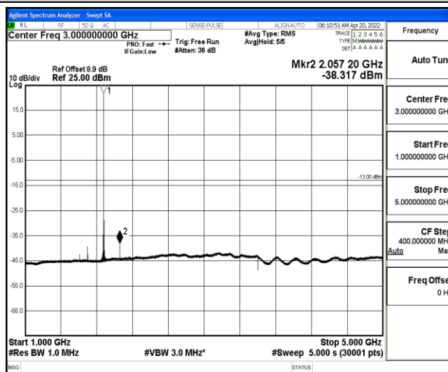
Band25-10MHz-16QAM-26365-1-0-Low-1000-5000--38.32-PASS
