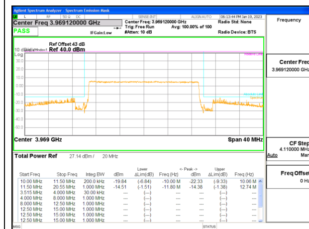
5G NR n77 20MHz QPSK High Channel
