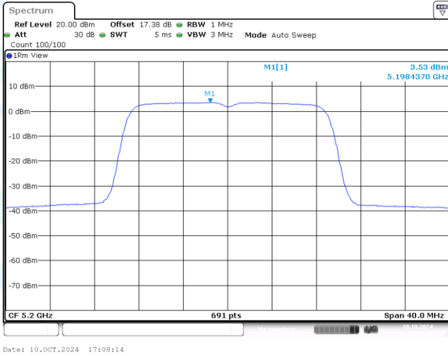
11N20MIMO-Ant1-5200-PASS
