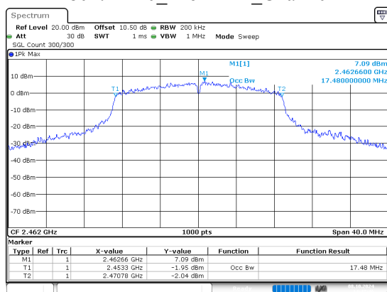
802.11n20_2462MHz_Chain 0
