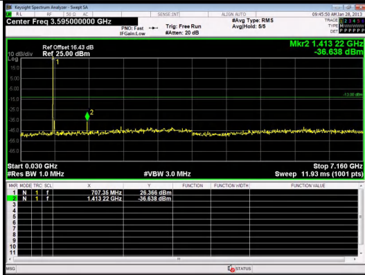
30.0MHz-7160.0MHz Band 12 3MHz/707.5/Mid QPSK 1@0
