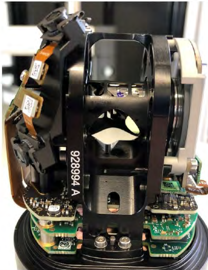
Subassembly-Lidar_FronView_Mirror
