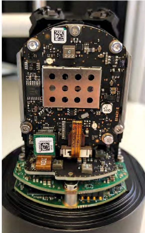
Subassembly-Lidar_EDMPCBA_Tx
