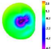
2500.000MHz E1
