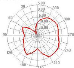
2400.000MHz E1
