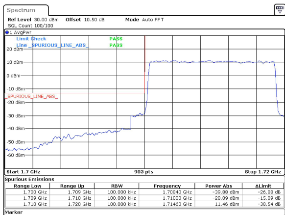
10MHz_15kHz_1715MHz_DFT-s-OFDM QPSK_RB50@0&-28.09 dBm
