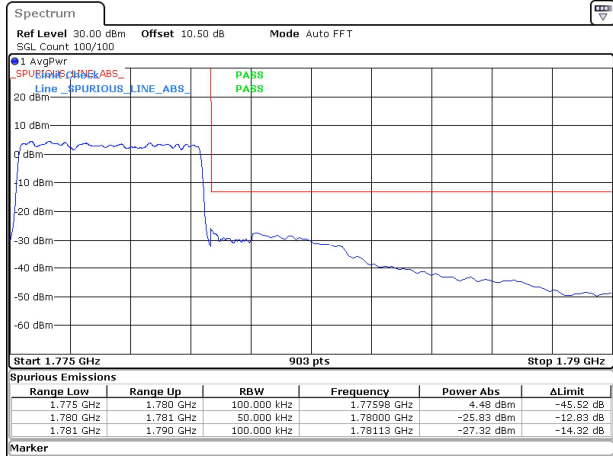
5MHz_15kHz_1777.5MHz_DFT-s-OFDM QPSK_RB25@0&-25.83 dBm
