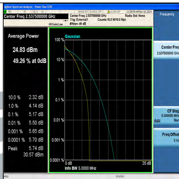
Band41(2535-2655)-5MHz-QPSK-40065-25RB#0-PASS
