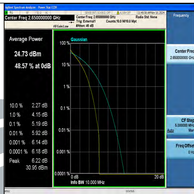
Band41(2535-2655)-10MHz-QPSK-41190-50RB#0-PASS
