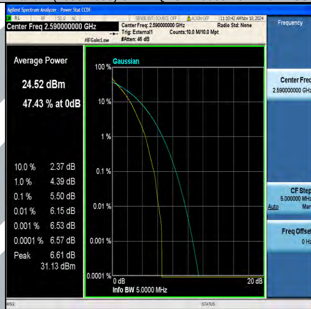
Band41(2535-2655)-5MHz-QPSK-40590-25RB#0-PASS
