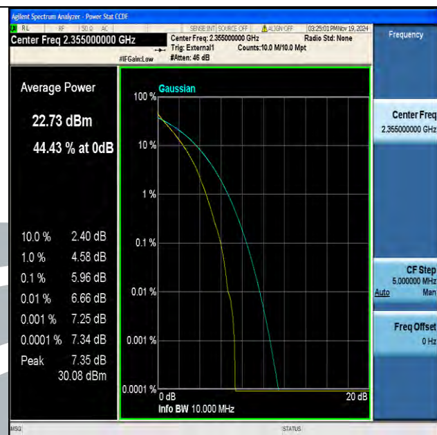
Band40(2350-2360)-10MHz-QPSK-39200-50RB#0-PASS
