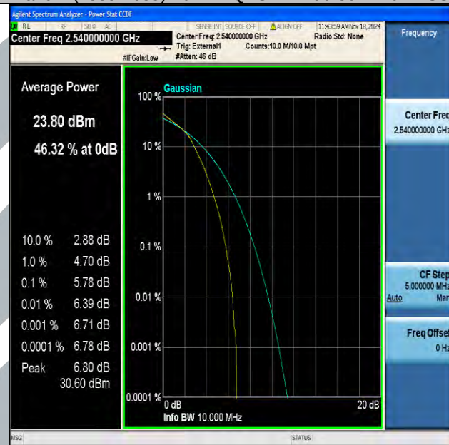
Band41(2535-2655)-10MHz-16QAM-40090-50RB#0-PASS
