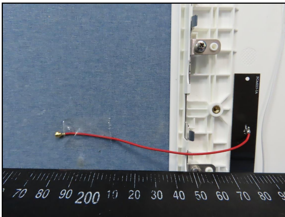
GPS(L1) Antenna
