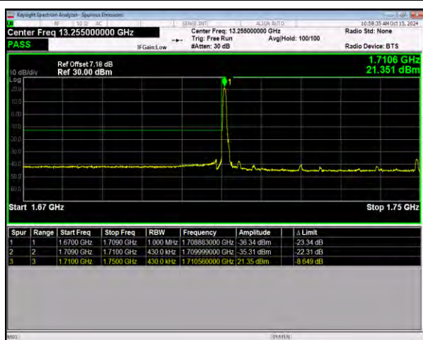
n66 SCS=15kHz DFT_16QAM BW=40MHz LowChannel=346000 RB=1@0
