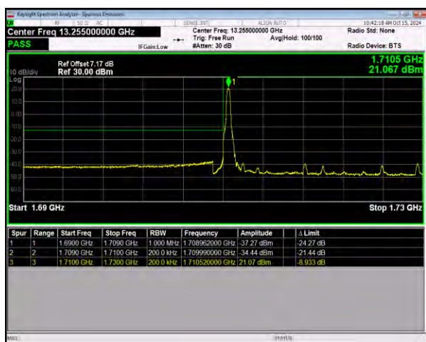
n66 SCS=15kHz DFT_QPSK BW=20MHz LowChannel=344000 RB=1@0
