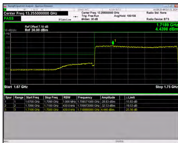
n66 SCS=15kHz DFT_QPSK BW=40MHz LowChannel=346000 RB=216@0
