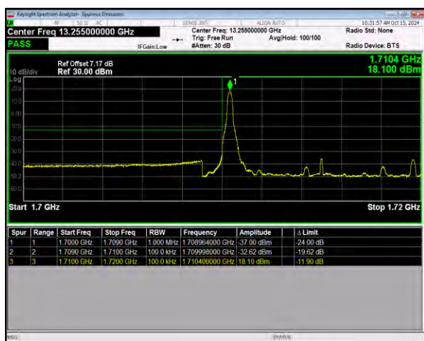
n66 SCS=15kHz DFT_16QAM BW=10MHz LowChannel=343000 RB=1@0
