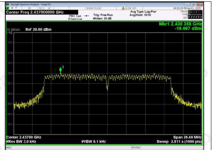
IEEE 802.11n_Channel 6_20MHz
