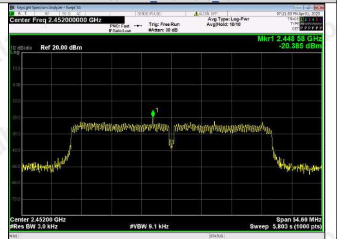
IEEE 802.11n_Channel 9_40MHz
