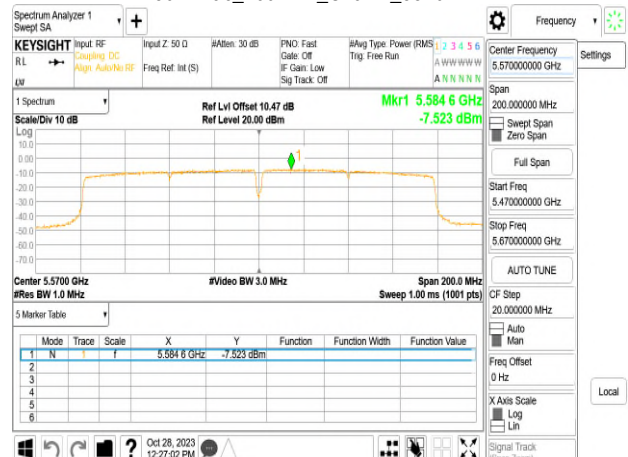
802.11ac_160MHz_Chain1_5570MHz
