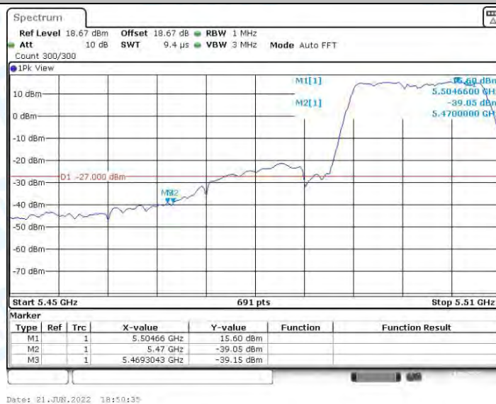
11A_Ant2_Low_5500
