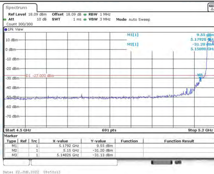
11N40MIMO_Ant2_Low_5190
