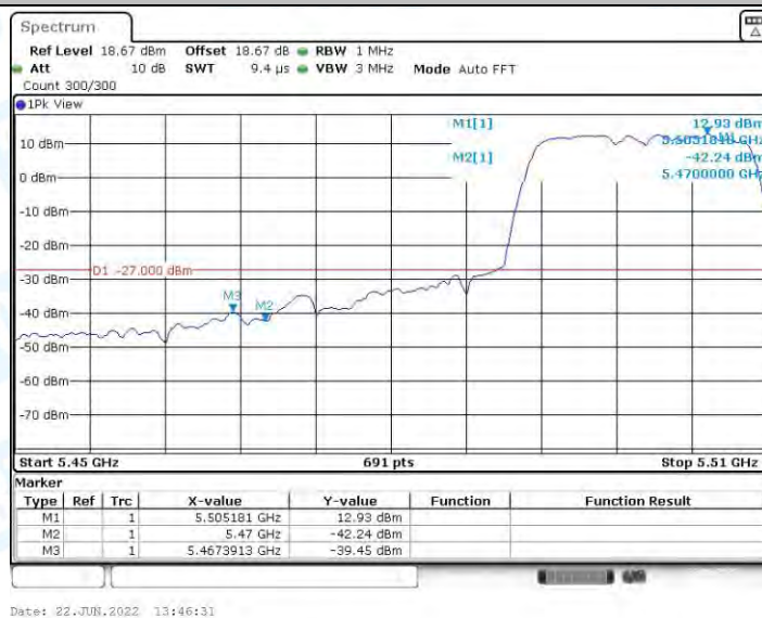
11AC20MIMO_Ant2_Low_5500
