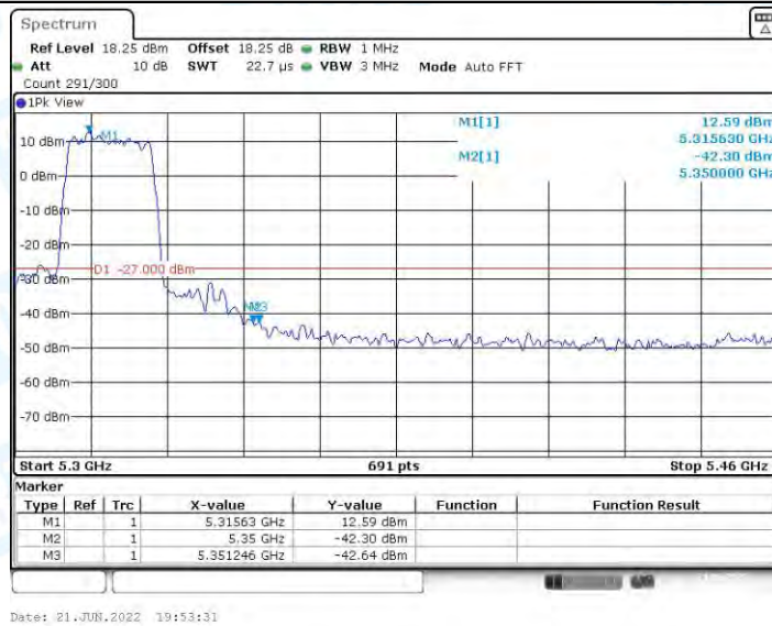
11N20MIMO_Ant2_High_5320
