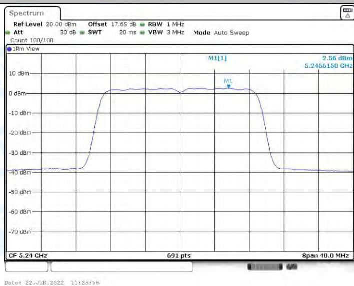
11AC20MIMO_Ant1_5240
