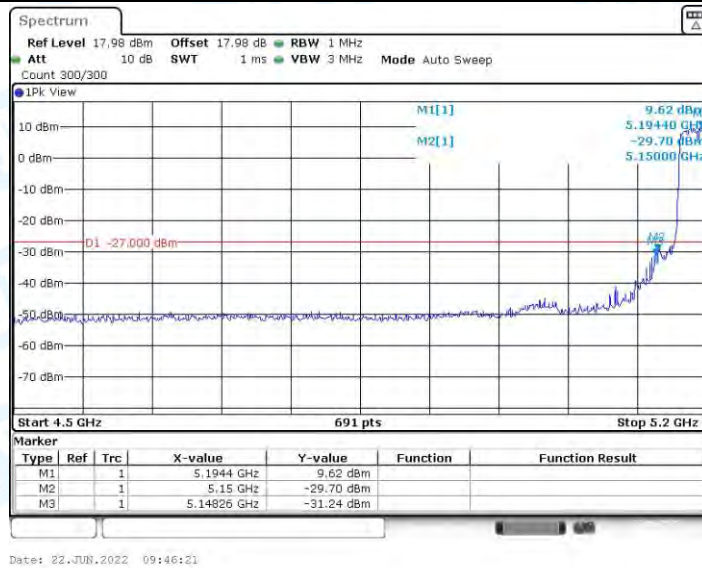
11N40MIMO_Ant1_Low_5190
