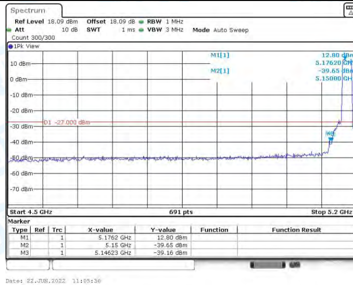
11AC20MIMO_Ant2_Low_5180
