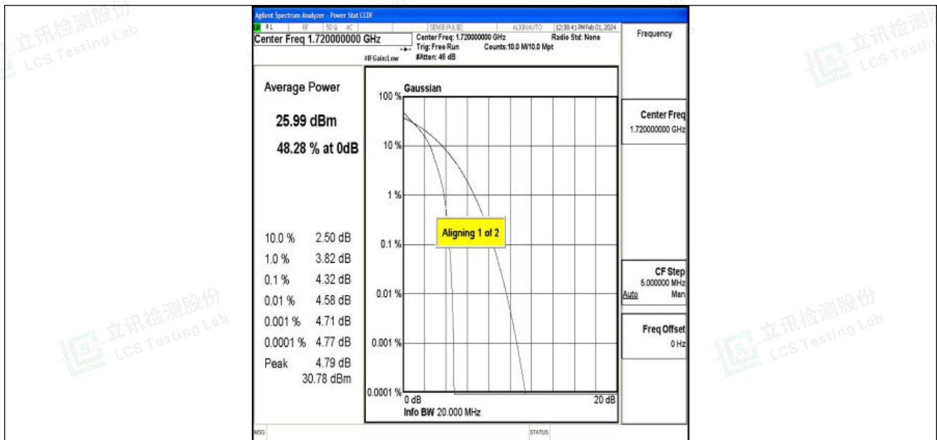
Band4-20MHz-QPSK-20050-1RB#0-PASS
