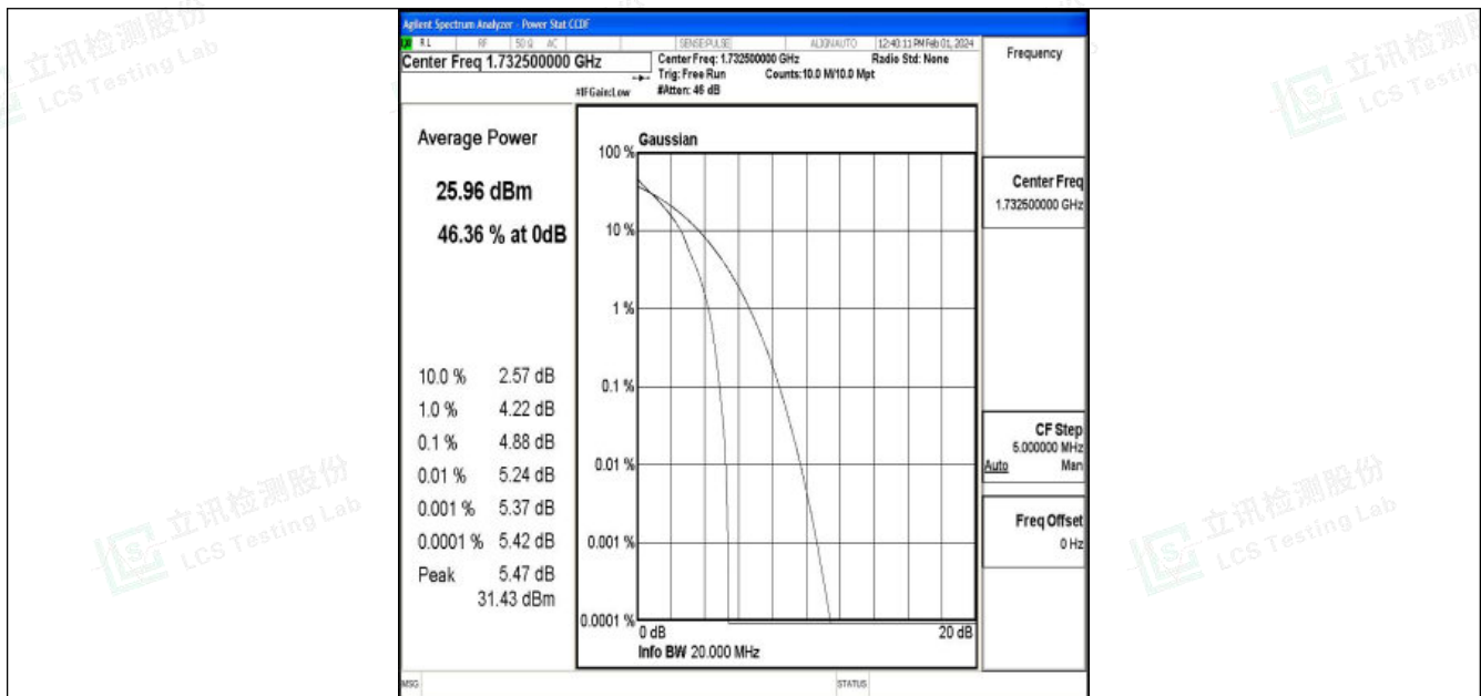
Band4-20MHz-QPSK-20175-1RB#0-PASS
