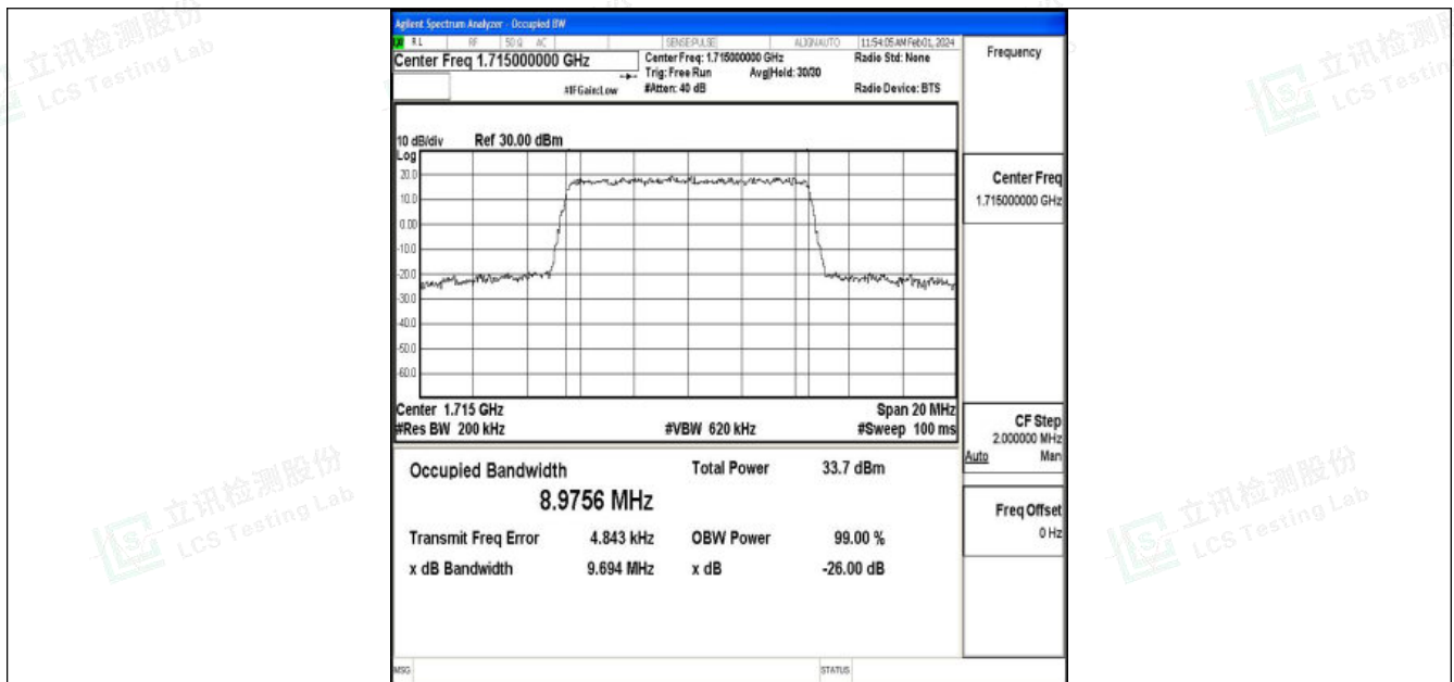
Band4-10MHz-QPSK-20000-50RB#0-PASS
