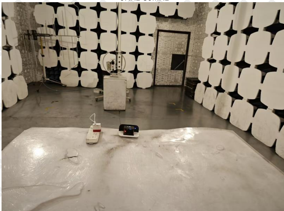
9KHz-30MHz
