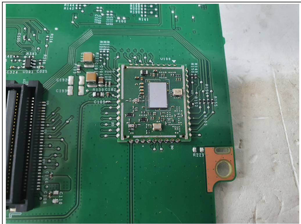
<WIFI, BT_Module>
