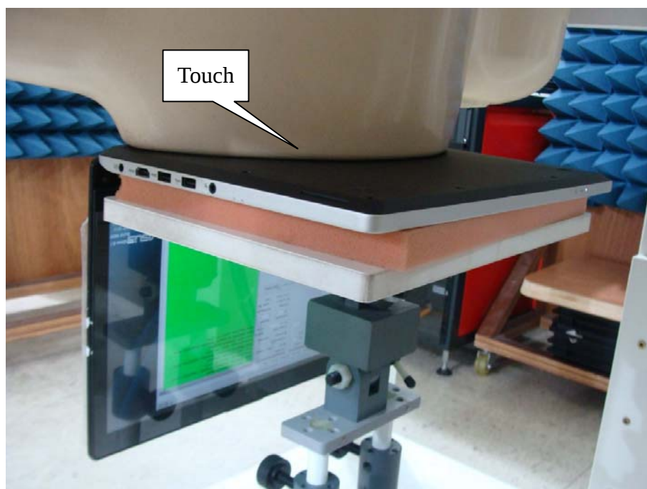
EUT Bottom (NB Mode)
