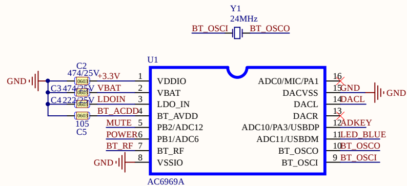
MCU: AC6969A
