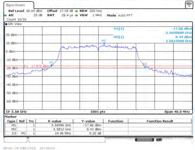
11A-Ant1-5580
