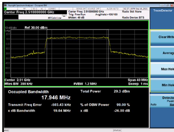
NR n7 16QAM 100%RB CH-Middle
