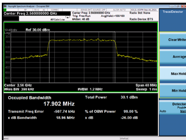
NR n7 P1/2 BPSK 100%RB CH-High
