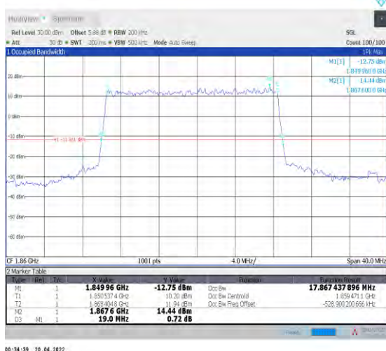
1-N25--15-20-L-2-DFT-PI2BPSK-Outer_Full-100@0-Ant 1-17.867-19.000-≤20-PASS
